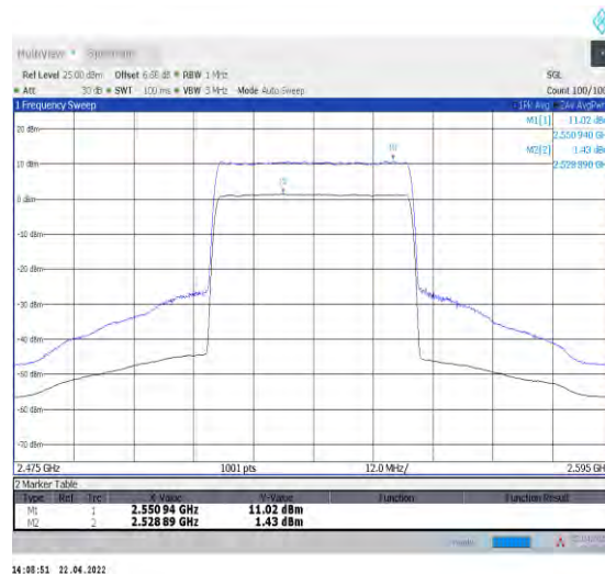
1-N7--15-40-M-2-CP-256QAM-Outer_Full-216@0-A nt0-9.59-100%-0.00-9.59-PASS-≤13
