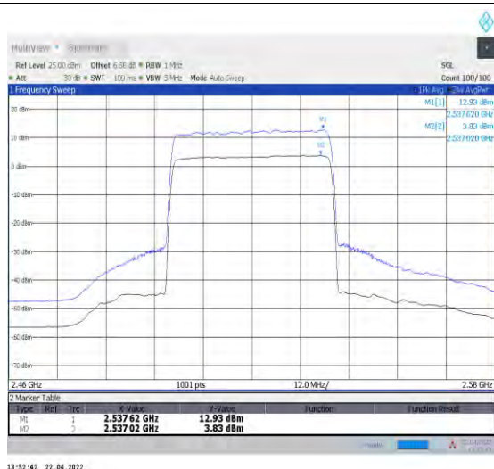
1-N7--15-40-L-1-DFT-256QAM-Outer_Full-216@0-A nt0-9.10-100%-0.00-9.10-PASS-≤13
