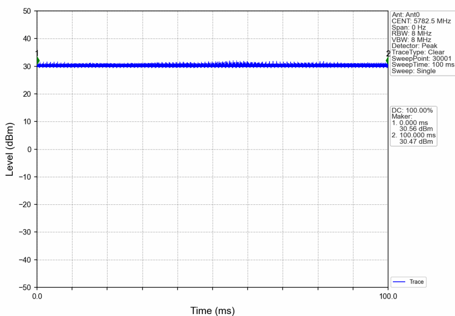
5M_MCH_5782.5MHz_Ant0_NTNV
