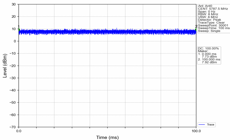
60M_MCH_5787.5MHz_Ant0_NTNV
