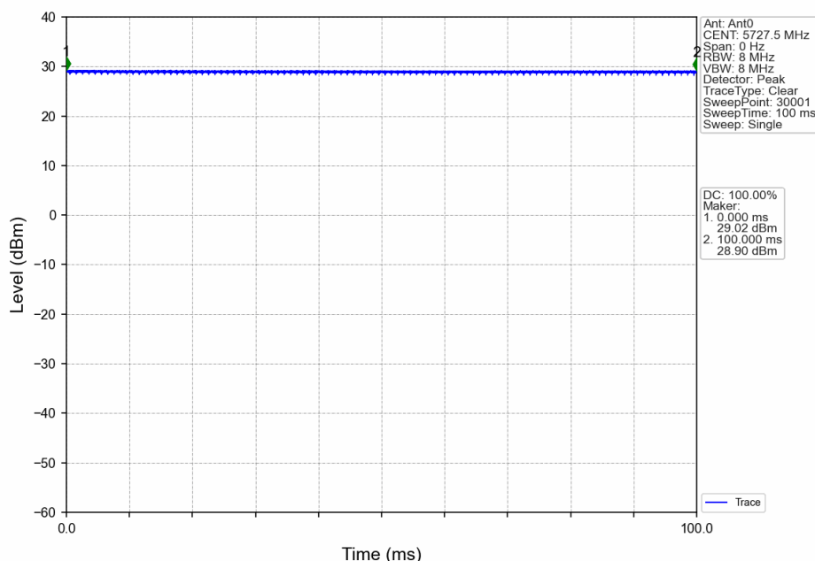
3M_LCH_5727.5MHz_Ant0_NTNV
