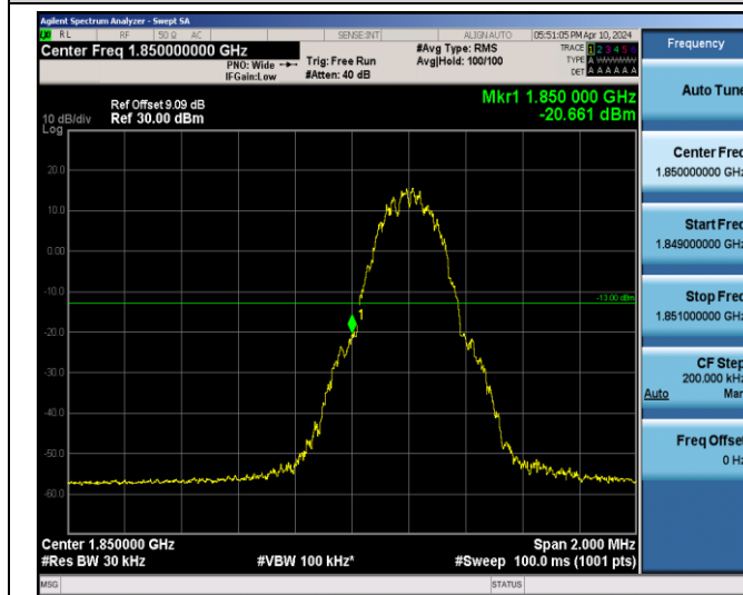
GSM1900-512-0
