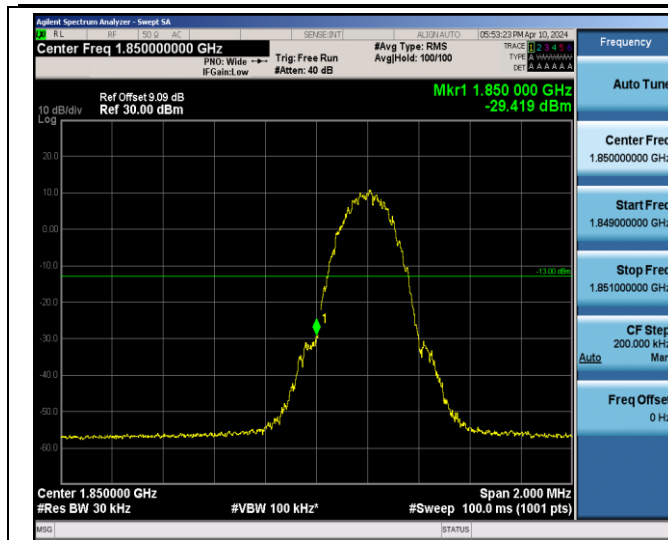
EGPRS1900-512-2
