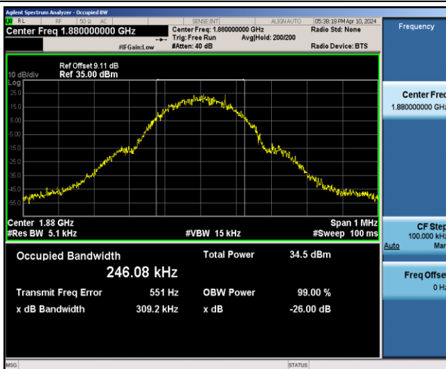
GSM1900-661-0-0.3092
