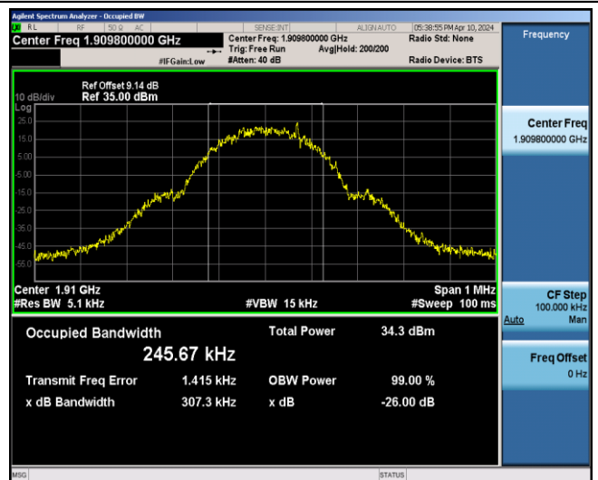
GSM1900-810-0-0.3073
