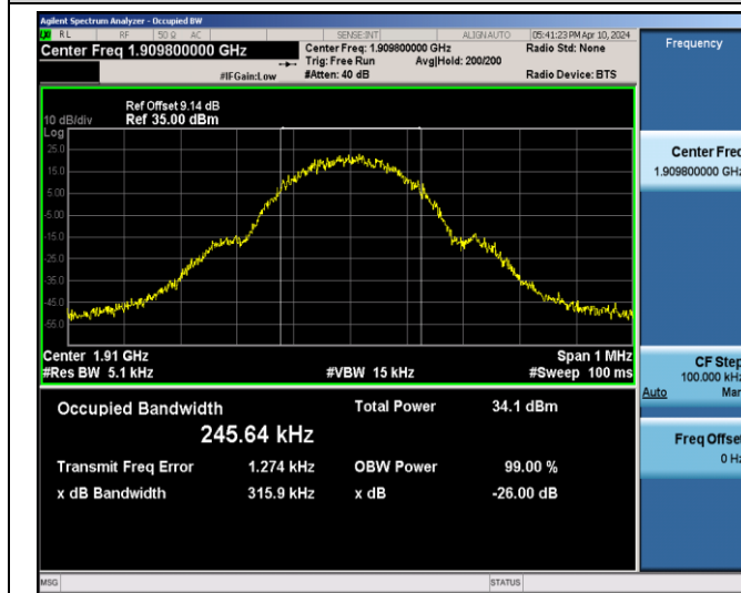
GPRS1900-810-0-0.3159
