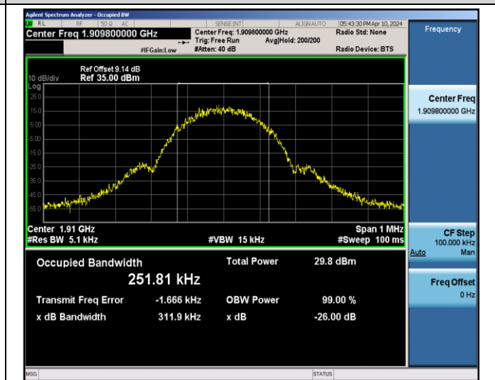
EGPRS1900-810-2-0.3119
