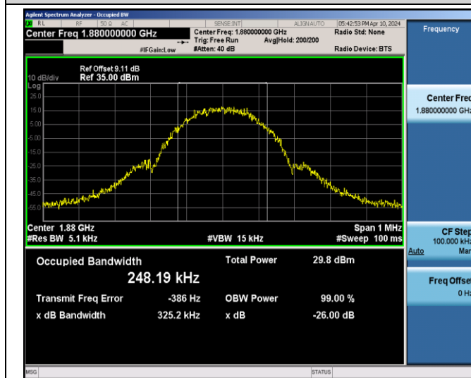
EGPRS1900-661-2-0.3252
