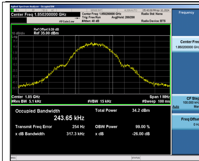
GPRS1900-512-0-0.3173
