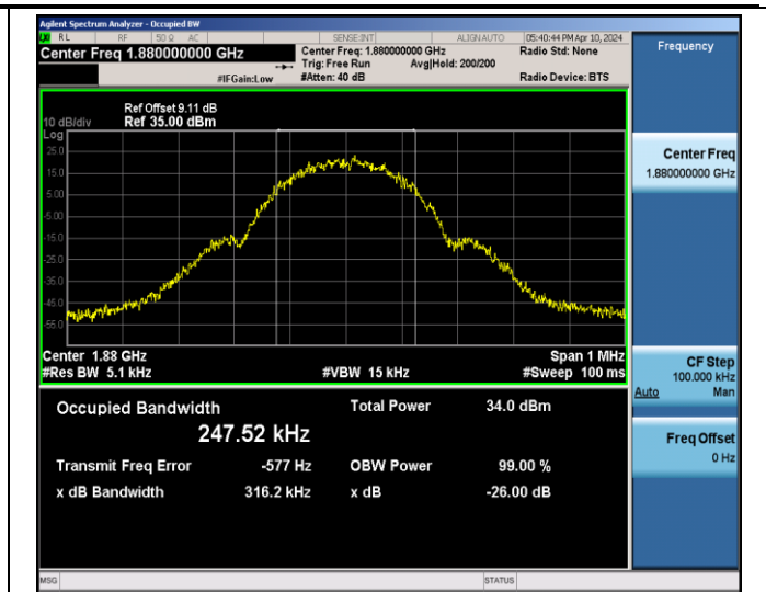
GPRS1900-661-0-0.3162
