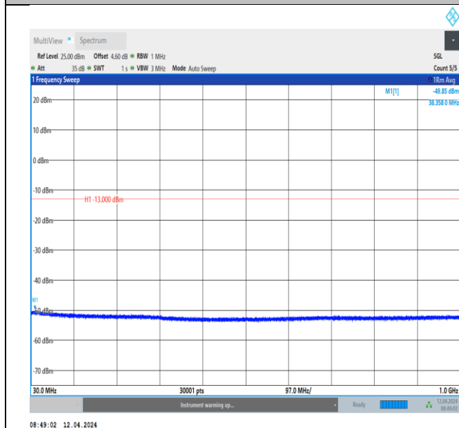
GSM1900-512-0-30~1000MHz-PASS
