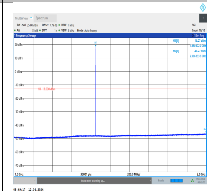
GSM1900-512-0-1000~3000MHz-PASS
