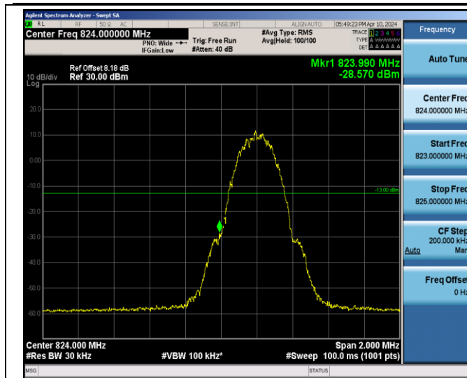
EGPRS850-128-8
