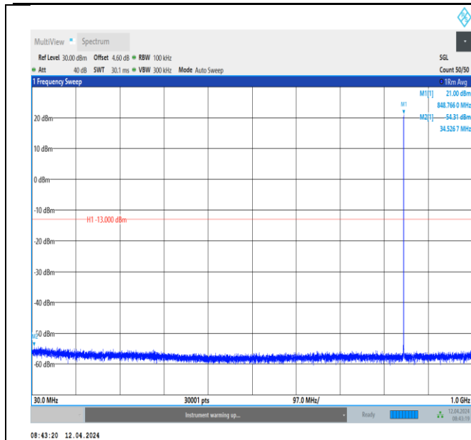
GSM850-251-5-30~1000MHz-PASS
