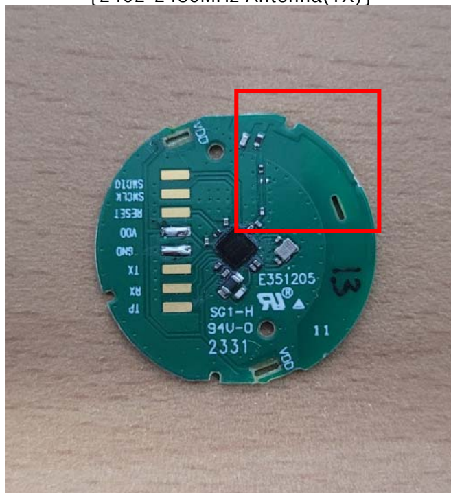
{ 2402-2480MHz Antenna(TX) }
