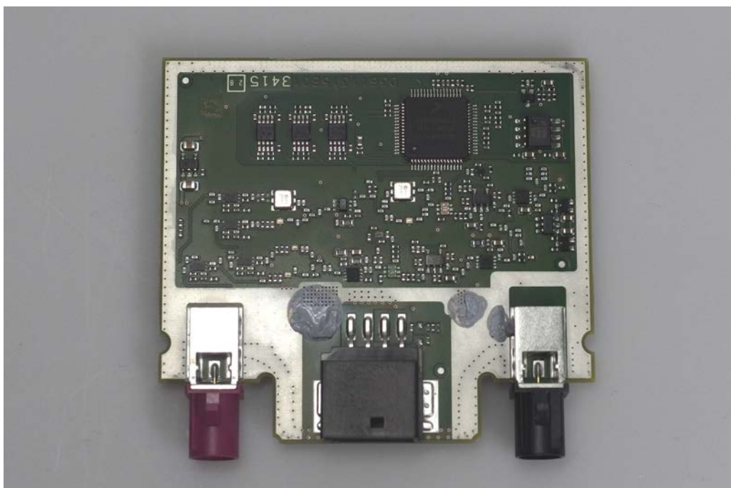
PCB Top Side:
