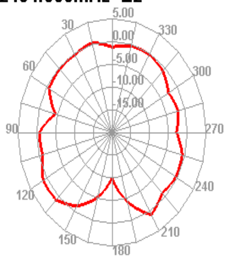
2484.000MHz E2
