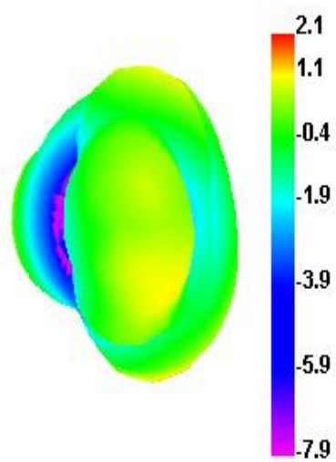
2441.000MHz
