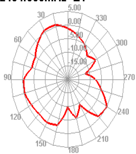
2484.000MHz E1
