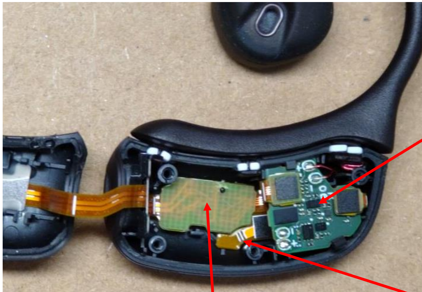
FPC
