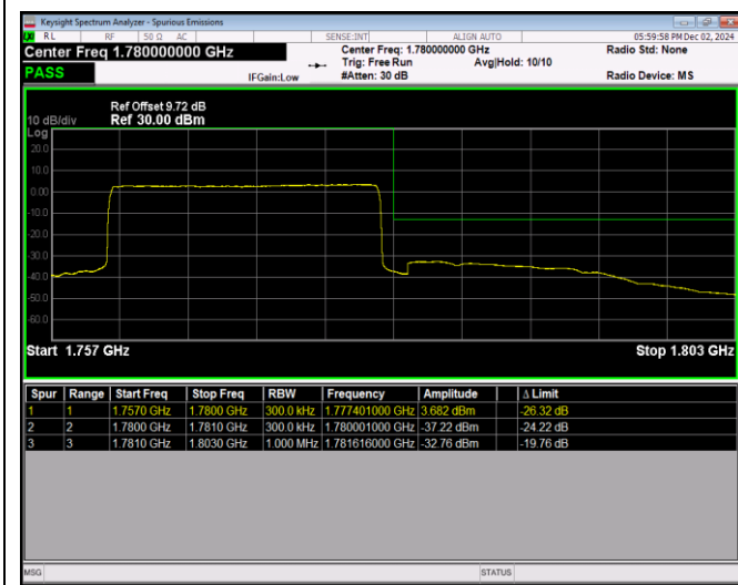
Band66-20MHz-16QAM-132072-1RB#99
