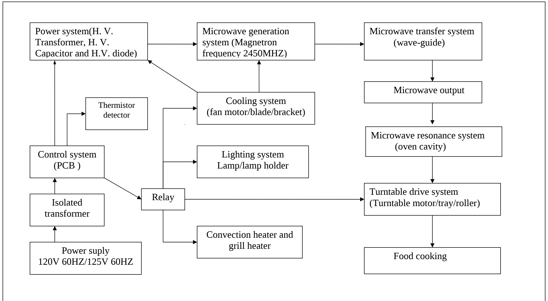
ED8525X-Y 产品方框图
