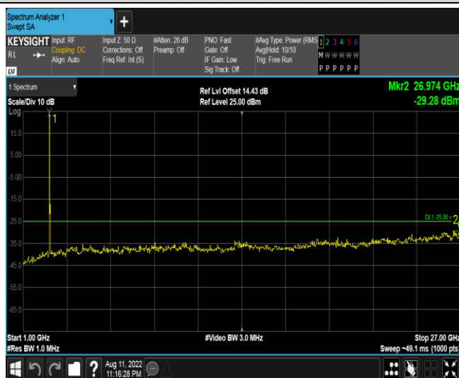
Band38-20MHz-16QAM-37850-1RB#0-Range2:1000~27000MHz
