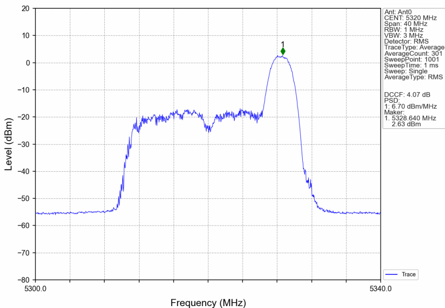
802.11ax(HEW20)_HCH_5320MHz_RU26_Right_Ant0_NTNV
