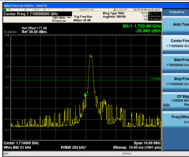
Band4-5MHz-QPSK-19975-1-0-Low--29.94-PASS
