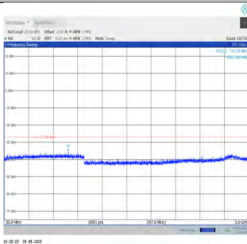
11ax40MIMO-Ant7-6525-30~3000
