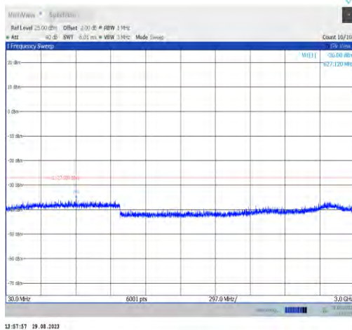
11ax40MIMO-Ant7-6685-30~3000
