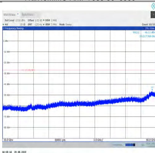
11ax40MIMO-Ant7-7085-10000~40000
