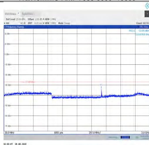
11ax40MIMO-Ant9-7085-30~3000
