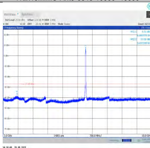
11ax40MIMO-Ant7-6885-3000~10000
