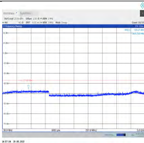
11ax40MIMO-Ant7-7085-30~3000
