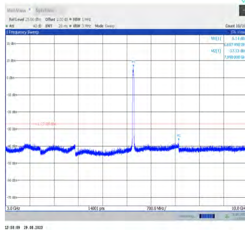
11ax40MIMO-Ant7-6685-3000~10000
