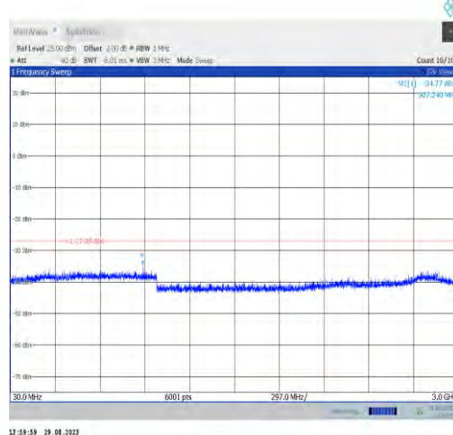
11ax40MIMO-Ant9-6685-30~3000
