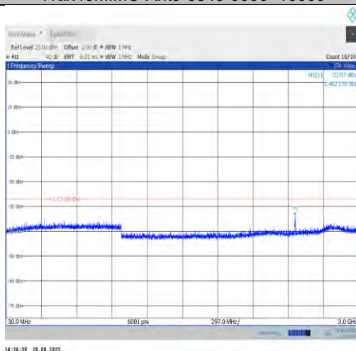
11ax40MIMO-Ant7-6885-30~3000
