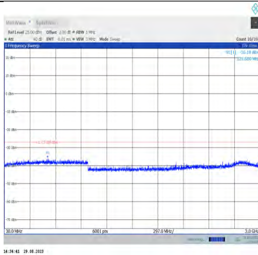
11ax40MIMO-Ant7-6925-30~3000
