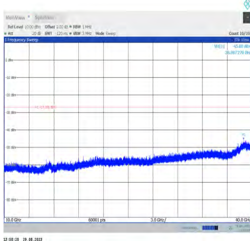
11ax40MIMO-Ant7-6685-10000~40000
