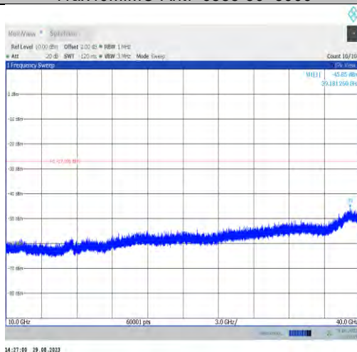
11ax40MIMO-Ant7-6885-10000~40000
