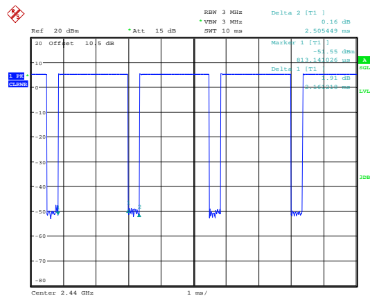
BLE 1Mbps Middle
