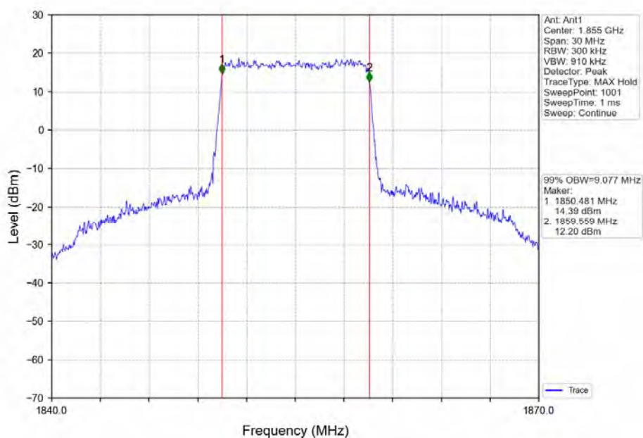
Band2_10MHz_QPSK_LCH_1855MHz_RB_50_0_NTNV
