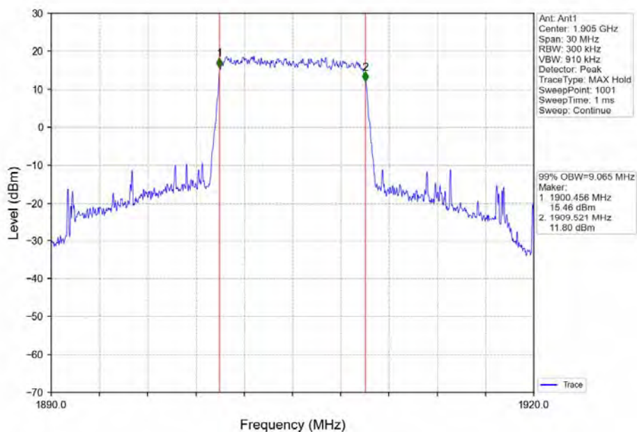
Band2_10MHz_QPSK_HCH_1905MHz_RB_50_0_NTNV
