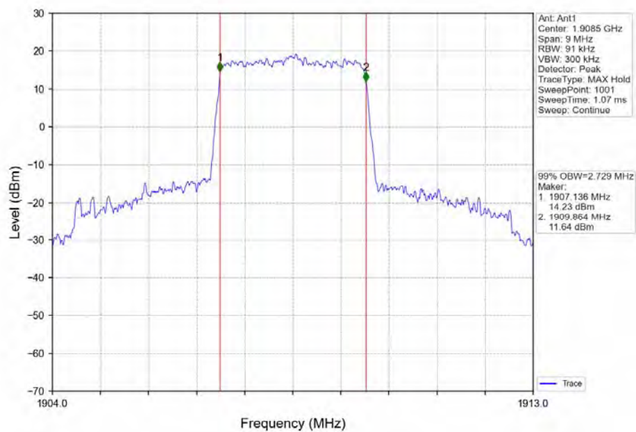
Band2_3MHz_QPSK_HCH_1908.5MHz_RB_15_0_NTNV
