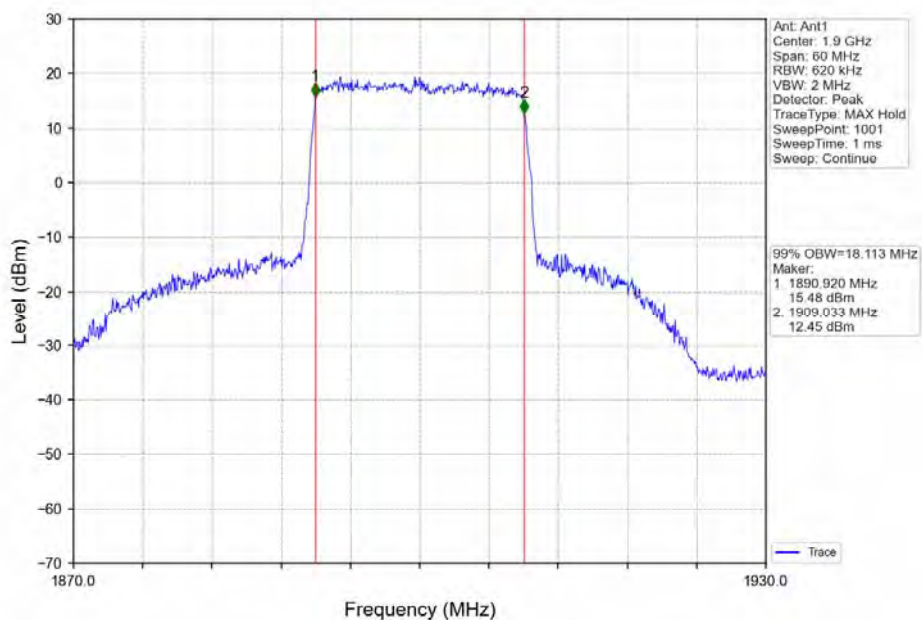
Band2_20MHz_QPSK_HCH_1900MHz_RB_100_0_NTNV
