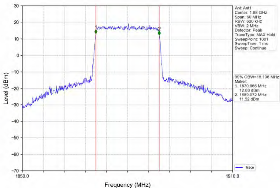
Band2_20MHz_16QAM_MCH_1880MHz_RB_100_0_NTNV
