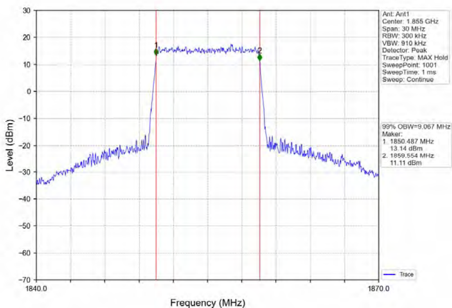
Band2_10MHz_64QAM_LCH_1855MHz_RB_50_0_NTNV
