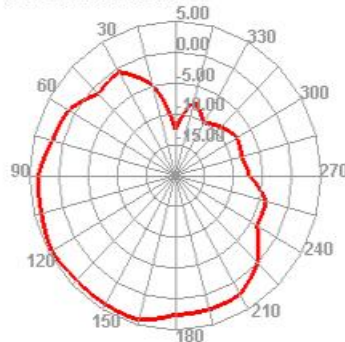
5500.000MHz H
