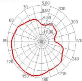
5850.000MHz H
