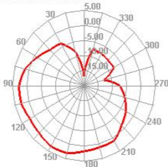
5150.000MHz H
