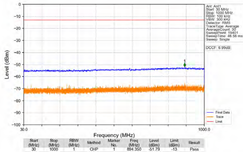
n77d_30kHz_SISO_NTNV_60MHz_DFT-s-OFDM_PI/2_BPSK_3480MHz_Edge_1RB_Left
