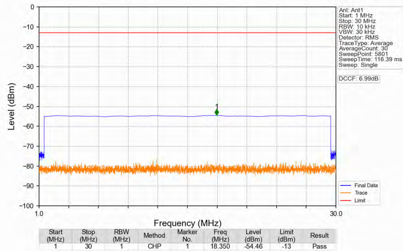
n77d_30kHz_SISO_NTNV_60MHz_DFT-s-OFDM_PI/2_BPSK_3480MHz_Edge_1RB_Left
