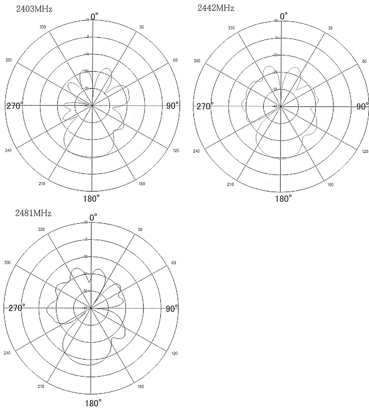
図 13 アンテナパターン図(垂直偏波、X軸回転)
