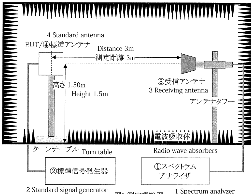
図1 測定概略図
