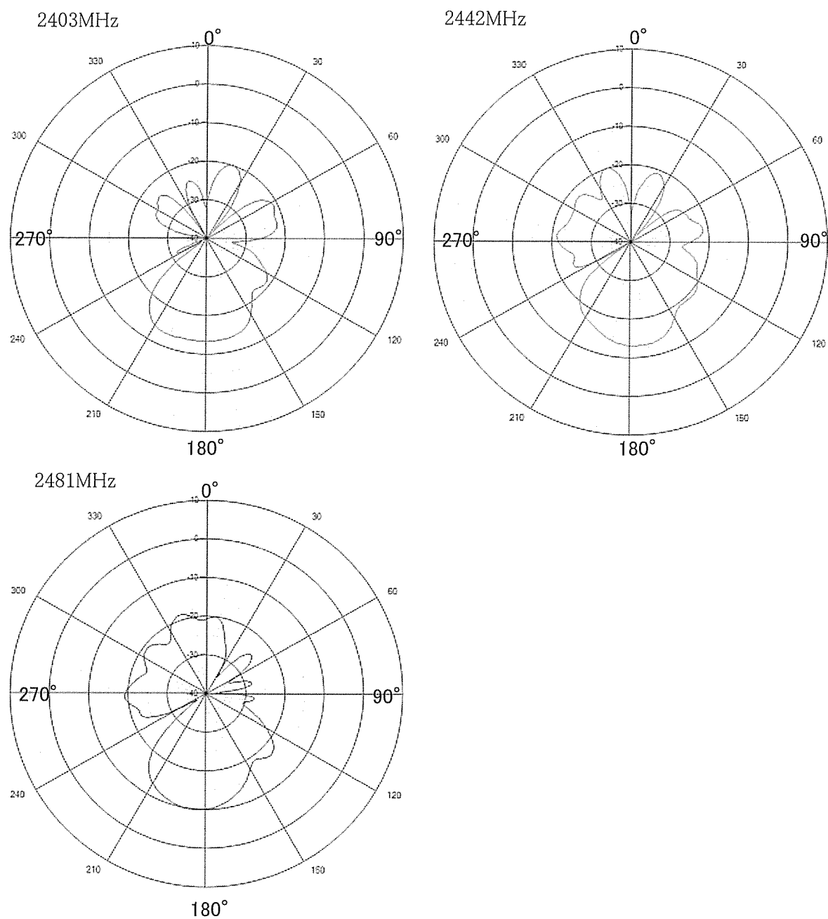
図 19 アンテナパターン図(垂直偏波、X軸回転)
