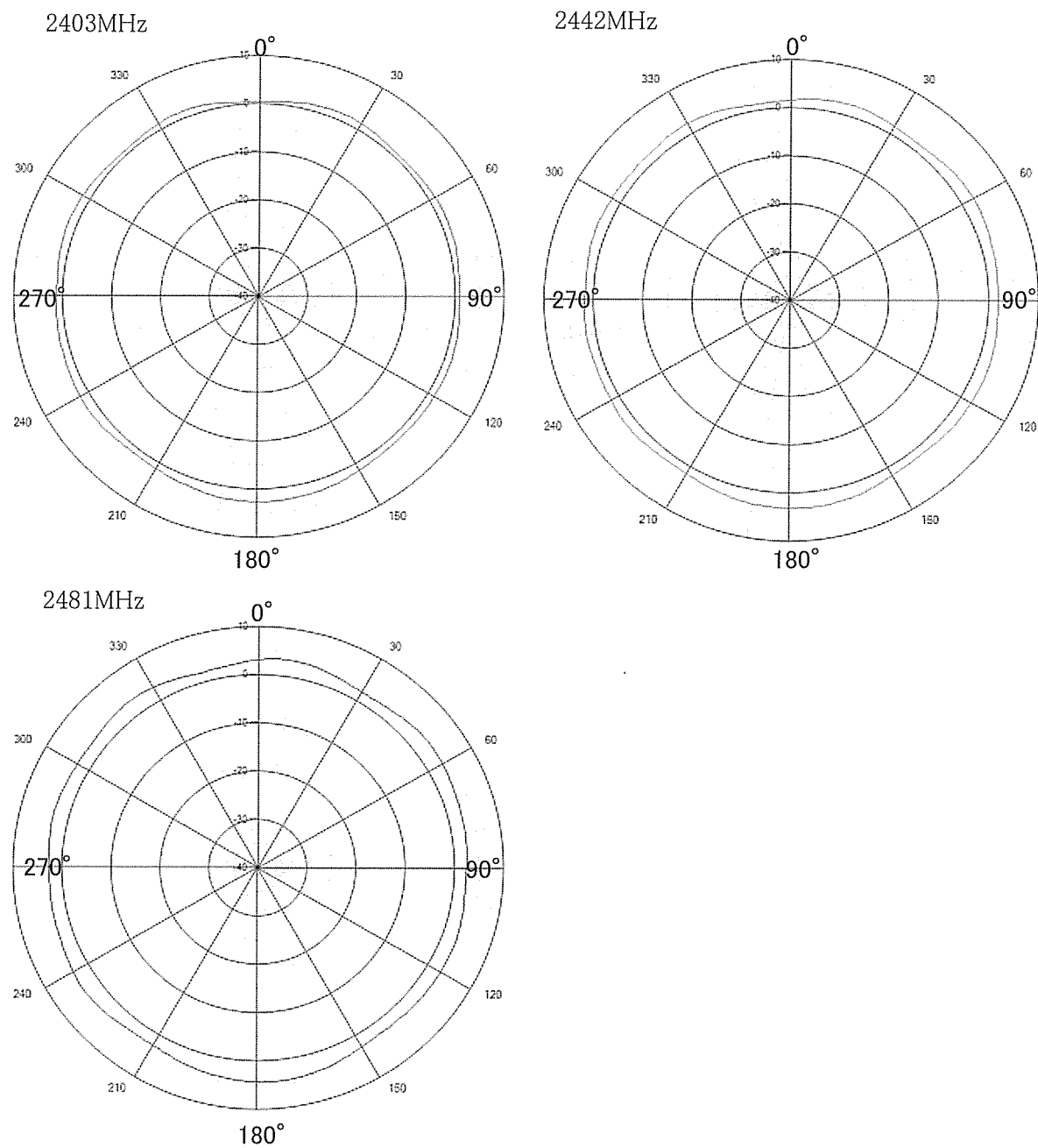
図 21 アンテナパターン図(垂直偏波、Y軸回転)
