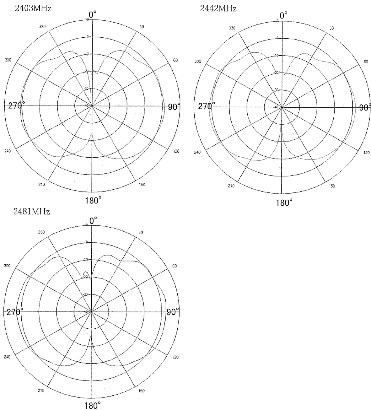
図 16 アンテナパターン図(水平偏波、Z軸回転)
