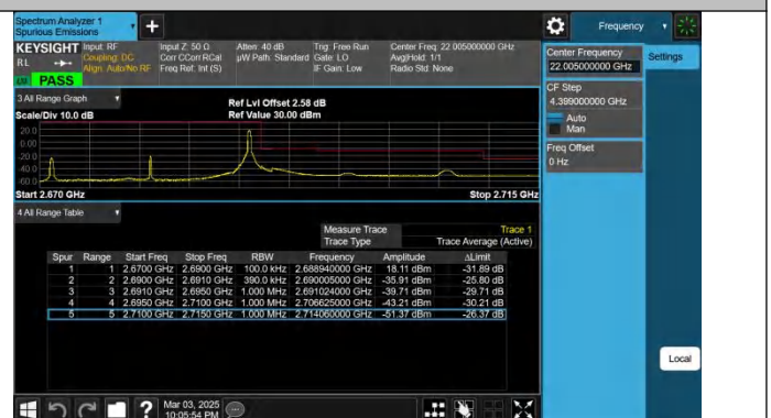
Band41-20MHz-QPSK-41490-1RB#99-PASS
