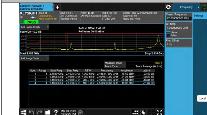
Band41-20MHz-QPSK-39750-1RB#99-PASS
