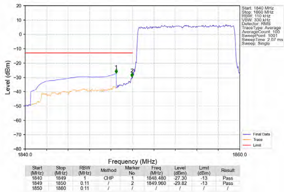
Band25_10MHz_QPSK_LCH_1855MHz_RB_50_0_NTNV
