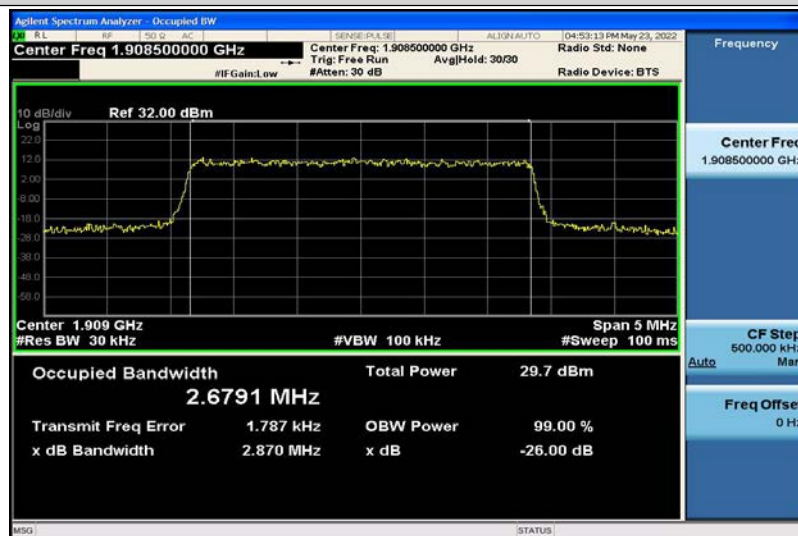
Band2-3MHz-QPSK-19185-15RB#0-2.6791
