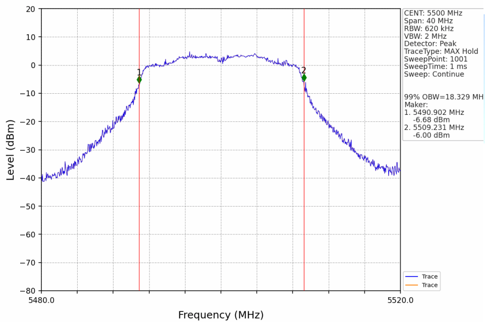
802.11ac(VHT20) LCH_5500MHz_Ant1_NTNV
