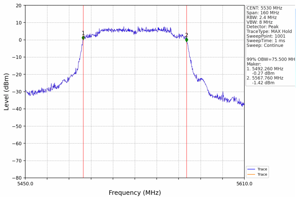
802.11ac(VHT80) LCH_5530MHz_Ant1_NTNV
