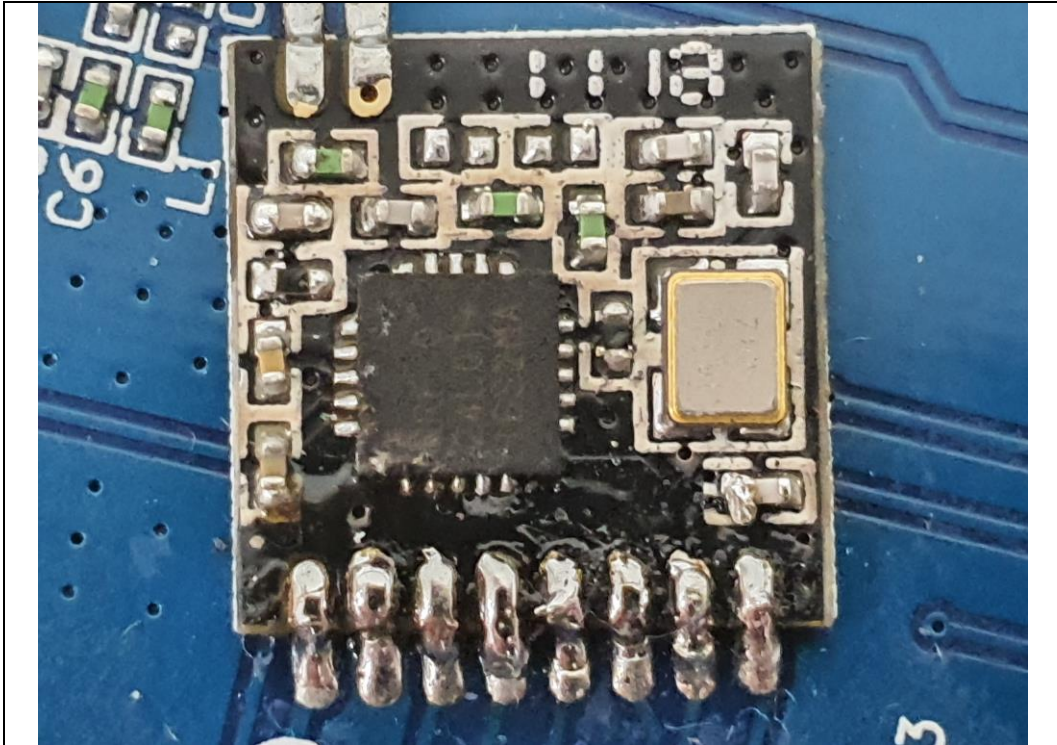
RF Module
