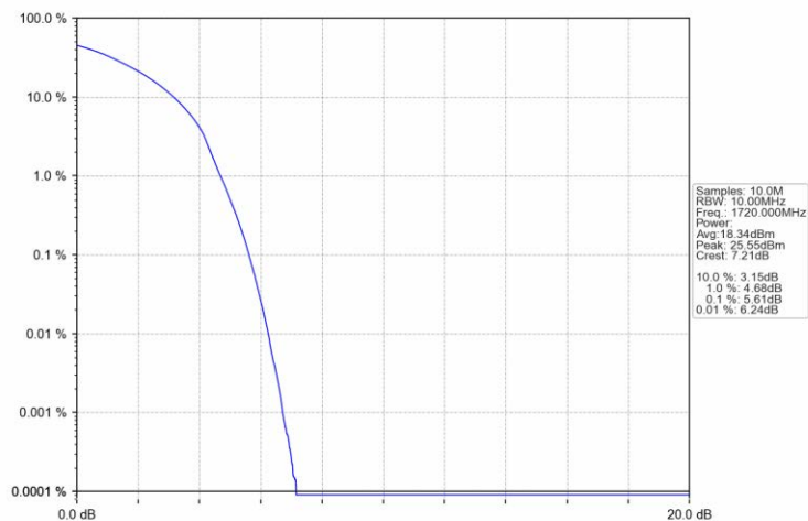
Band66 20MHz QPSK LCH 1720MHz RB 100 0 NTNV
