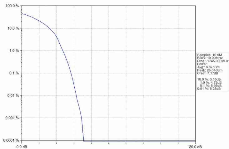
Band66 20MHz QPSK MCH 1745MHz RB 100 0 NTNV
