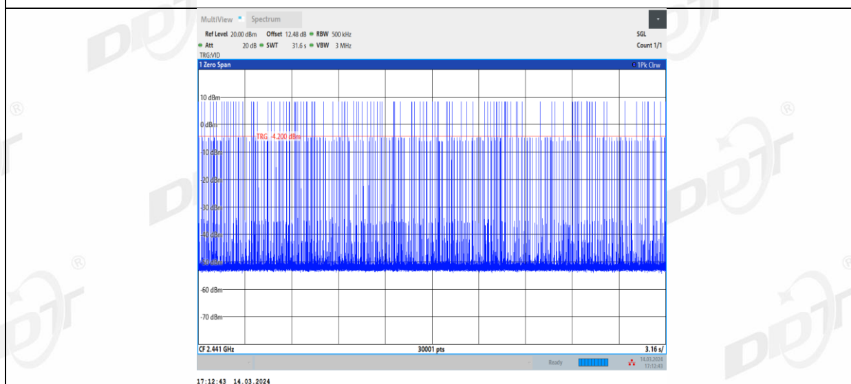
3DH3_Left side_Hop
