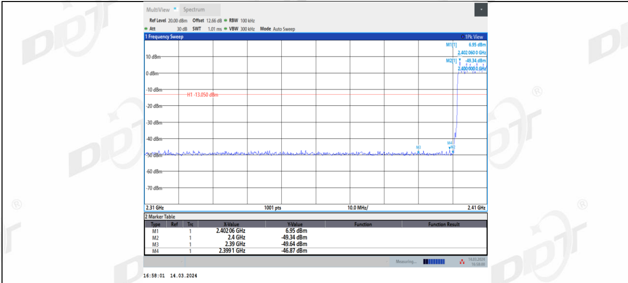
2DH5_Left side_Low_Hop_2402
