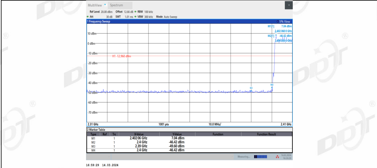
3DH5_Left side_Low_Hop_2402
