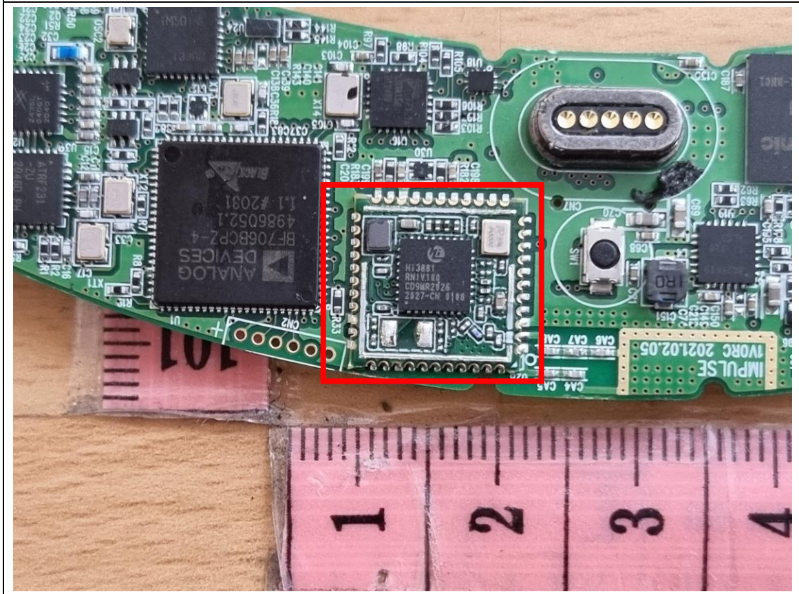
WLAN Module
