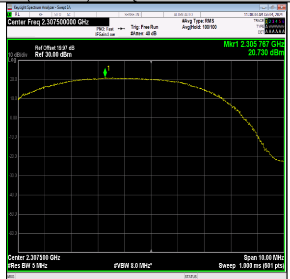
40(2305-2315)-5MHz-QPSK-38725-12RB#0-PASS
