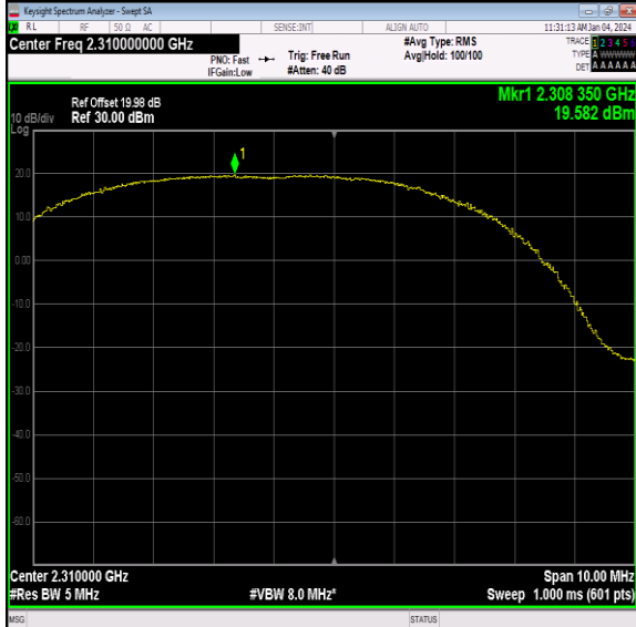
40(2305-2315)-5MHz-QPSK-38750-1RB#12-PASS
