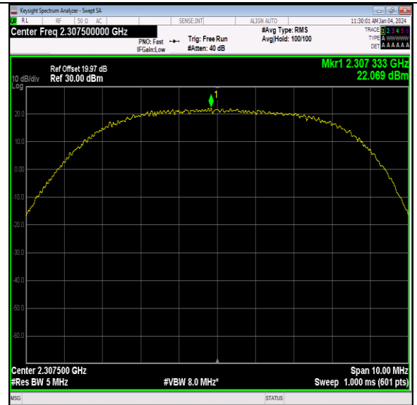
40(2305-2315)-5MHz-QPSK-38725-1RB#12-PASS
