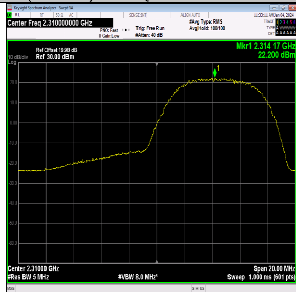
40(2305-2315)-10MHz-QPSK-38750-1RB#0-PASS
