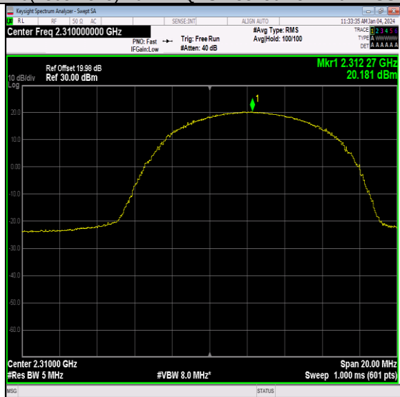
40(2305-2315)-10MHz-QPSK-38750-25RB#25-PASS
