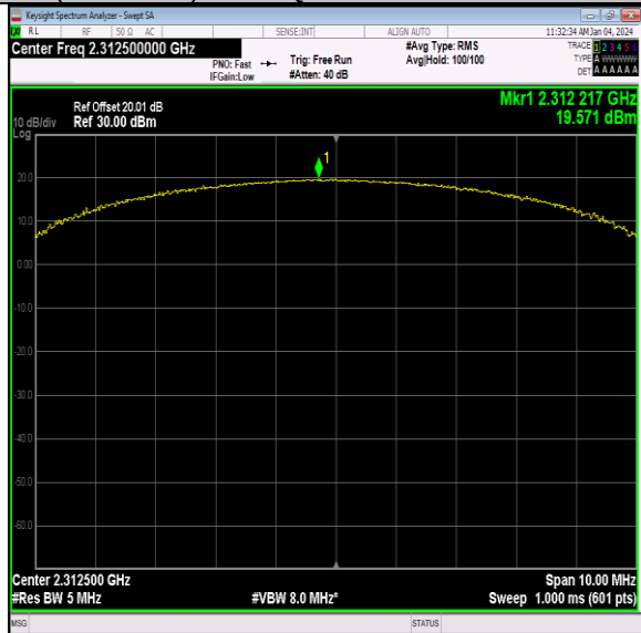
40(2305-2315)-5MHz-QPSK-38775-25RB#0-PASS
