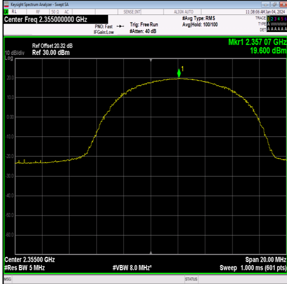
40(2350-2360)-10MHz-QPSK-39200-25RB#25-PASS
