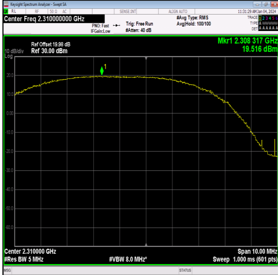
40(2305-2315)-5MHz-QPSK-38750-12RB#11-PASS
