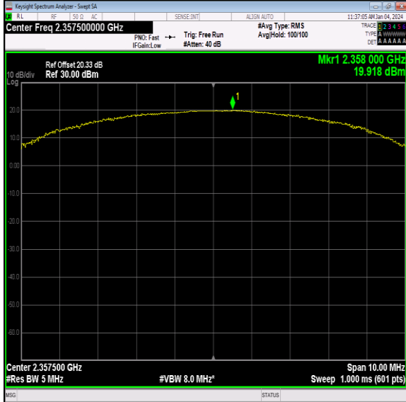
40(2350-2360)-5MHz-QPSK-39225-25RB#0-PASS
