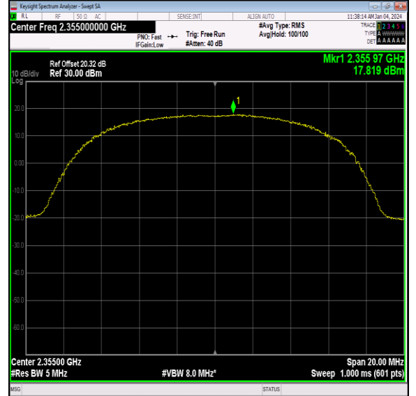
40(2350-2360)-10MHz-QPSK-39200-50RB#0-PASS
