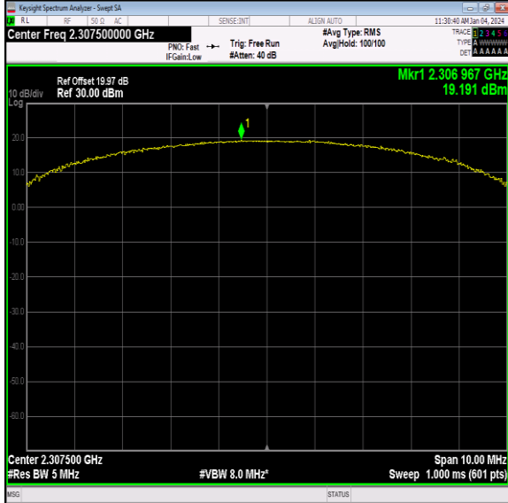
40(2305-2315)-5MHz-QPSK-38725-12RB#6-PASS
