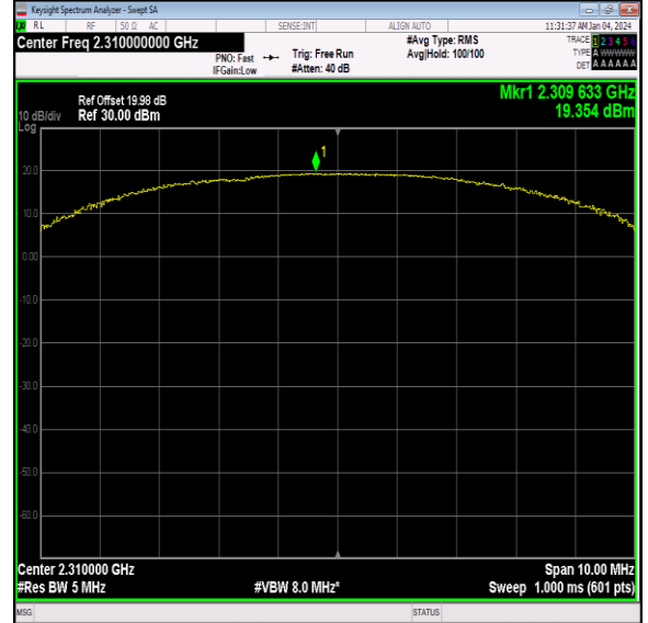
40(2305-2315)-5MHz-QPSK-38750-25RB#0-PASS
