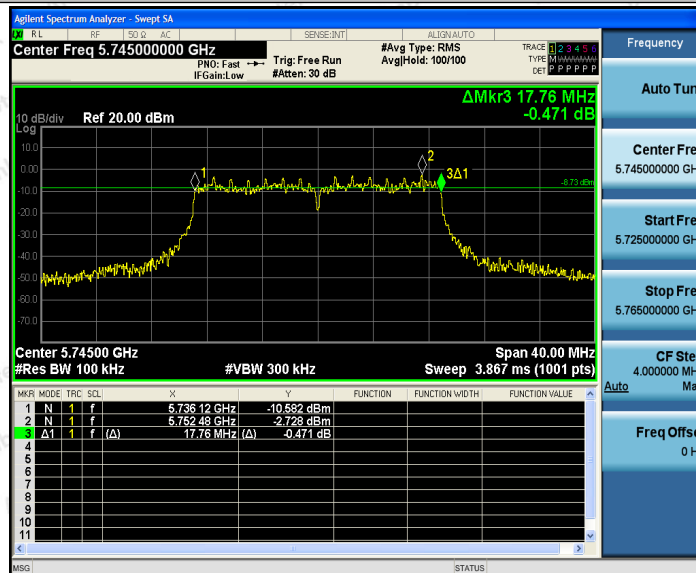
11N20SISO_Ant2_5745
