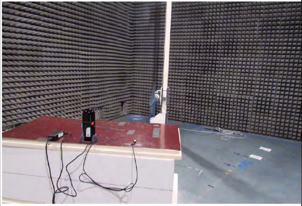
Setup 200 - 1000MHz
