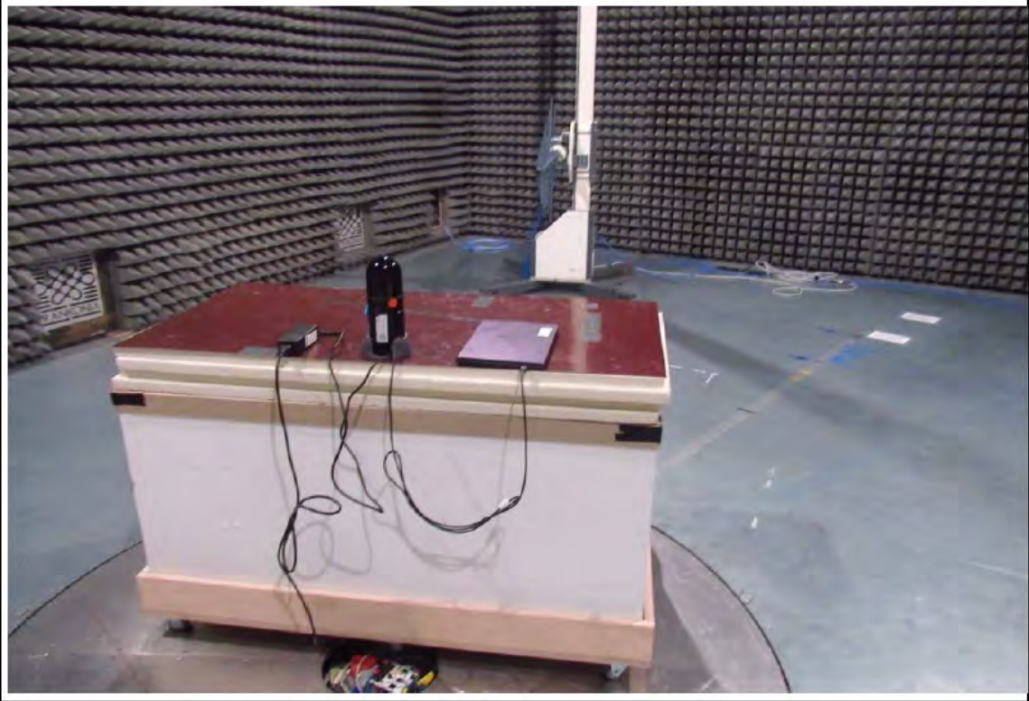
Setup 200 - 1000MHz
