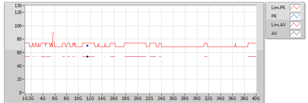
RE TX above 1GHz;Band:5.8G;VHT20,BF;BWch:20MHz;Nss:1,(M0);Nant:2;Ch:5745MHz;TX
