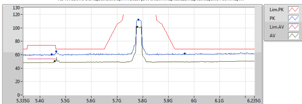
RE TX above 1GHz;Band:5.8G;VHT20,BF;BWch:20MHz;Nss:1,(M0);Nant:2;Ch:5785MHz;TX
