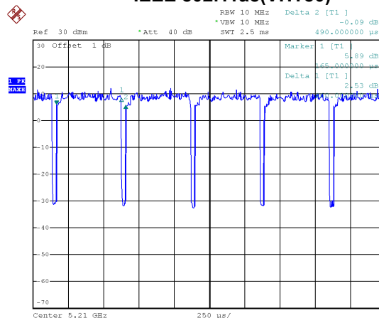
IEEE 802.11ac(VHT80)
