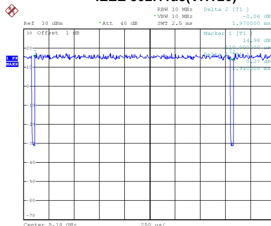
IEEE 802.11ac(VHT20)
