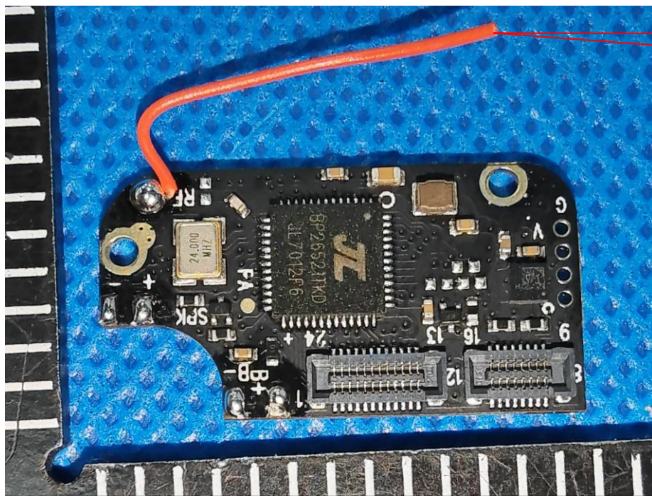
Antenna
