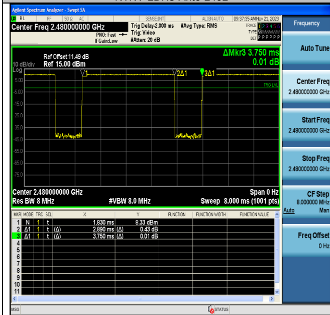
NTNV-2DH5-Ant6-2480
