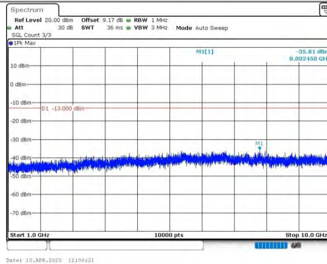
Band26@22-5MHz-QPSK-26715-1RB#0-Range2:1000~10000MHz
