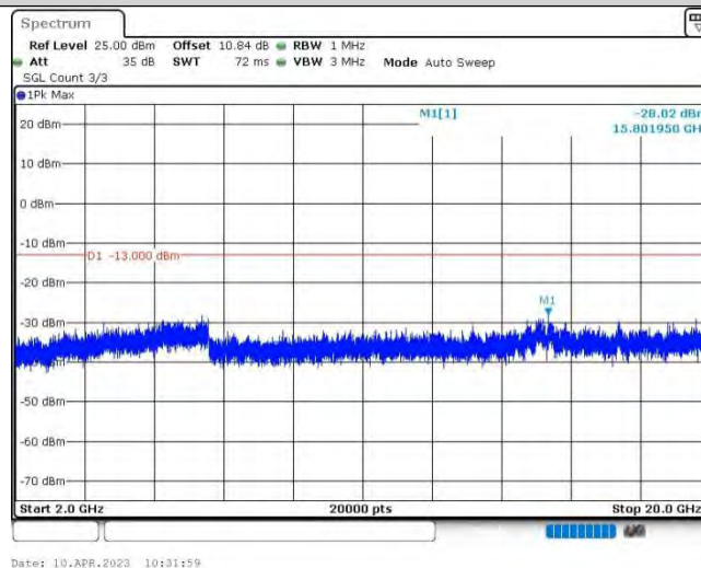
Band25-3MHz-QPSK-26365-1RB#0-Range3:2000~20000MHz
