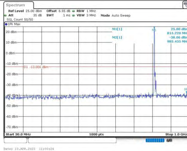
Band26@22-5MHz-QPSK-26715-1RB#0-Range1:30~1000MHz
