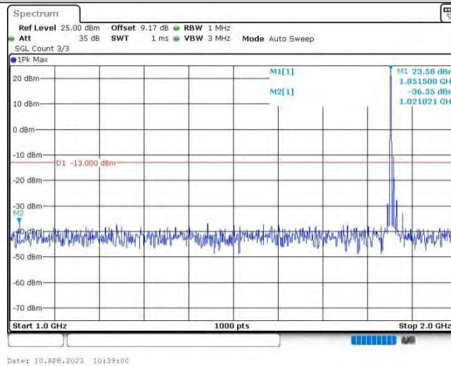
Band25-15MHz-QPSK-26115-1RB#0-Range2:1000~2000MHz
