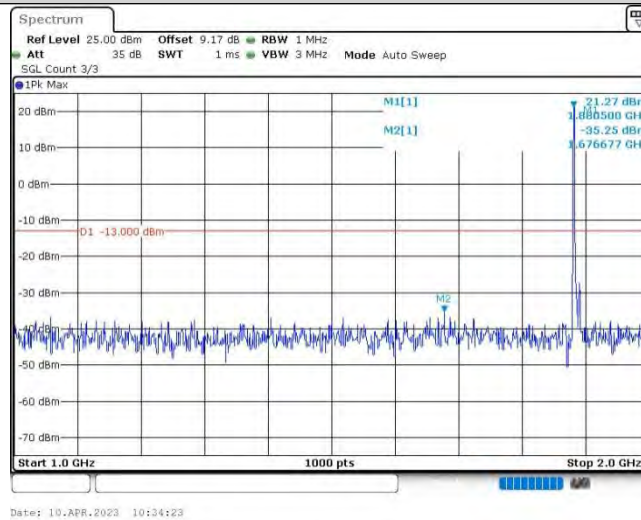
Band25-5MHz-QPSK-26365-1RB#0-Range2:1000~2000MHz
