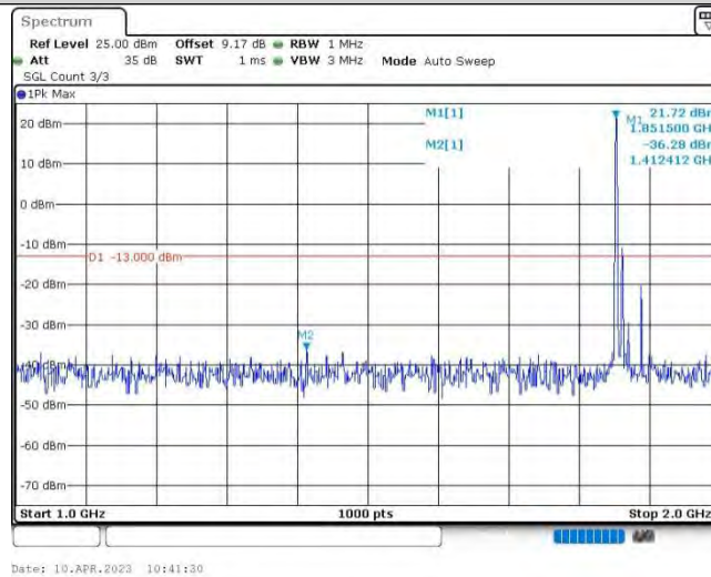
Band25-20MHz-QPSK-26140-1RB#0-Range2:1000~2000MHz
