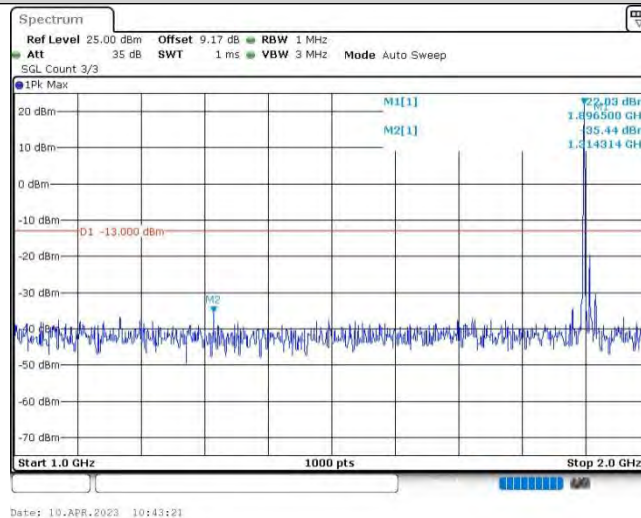
Band25-20MHz-QPSK-26590-1RB#0-Range2:1000~2000MHz
