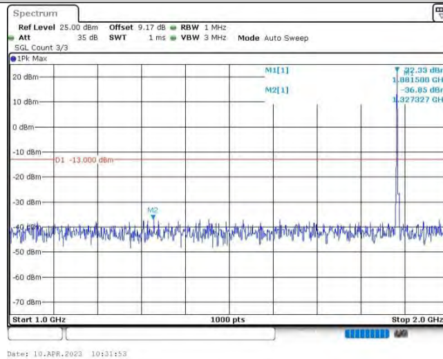
Band25-3MHz-QPSK-26365-1RB#0-Range2:1000~2000MHz
