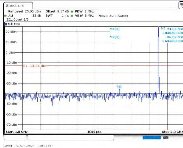
Band25-3MHz-QPSK-26055-1RB#0-Range2:1000~2000MHz
