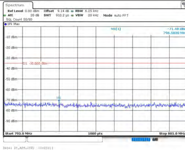
Band13-5MHz-QPSK-23230-1RB#0-Range2:793~805MHz
