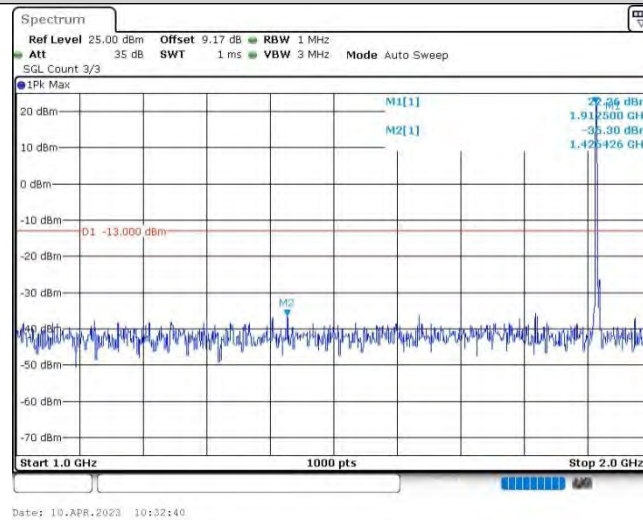
Band25-3MHz-QPSK-26675-1RB#0-Range2:1000~2000MHz
