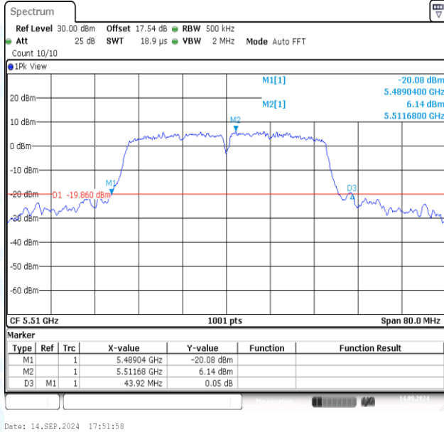
11N40MIMO-Ant1-5510
