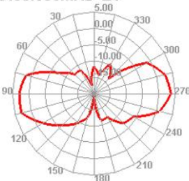
2450.000MHz E1
