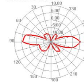
5500.000MHz E2
