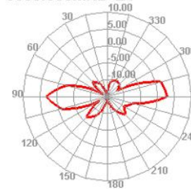
5500.000MHz E1
