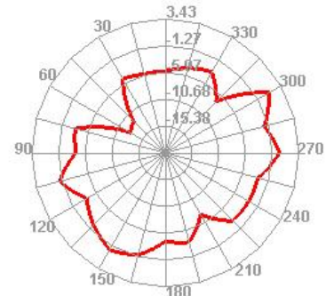
2450.000MHz E2
