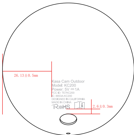
尺寸图
