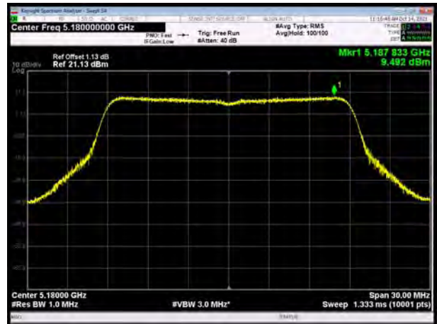
U-NII-1, 802.11n HT20
