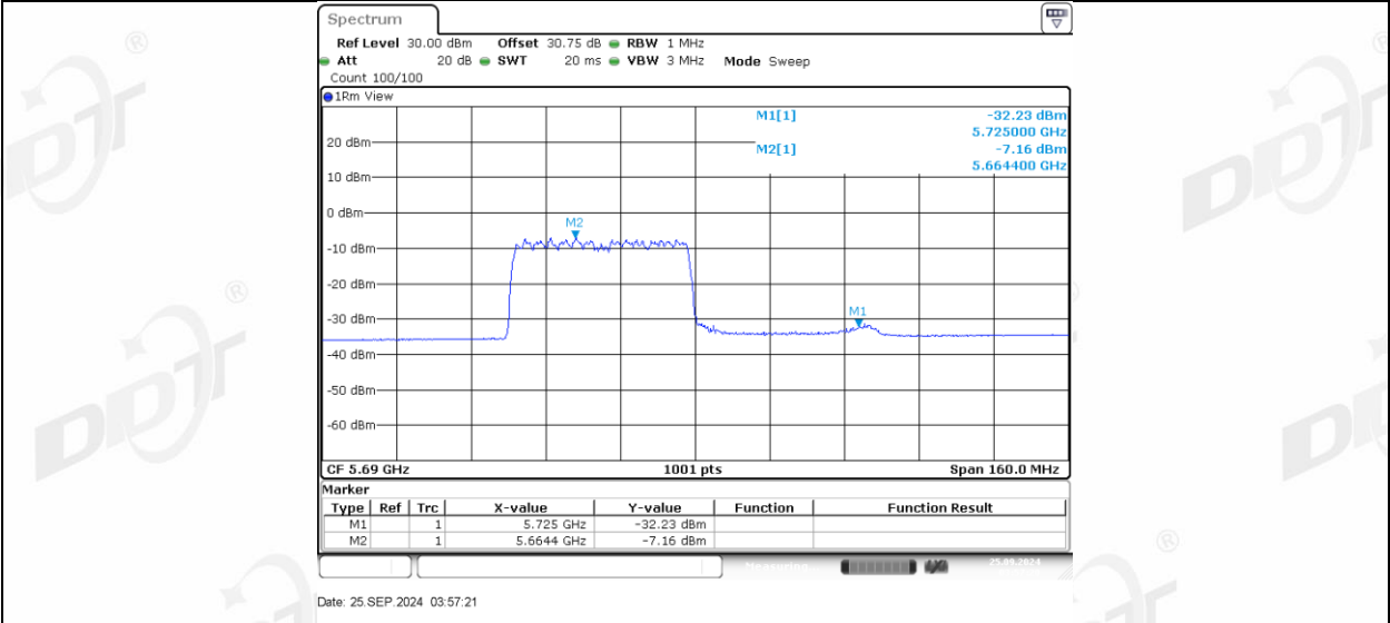
11AX80MIMO_Ant1_5690_UNII-2C_484Tone_RU66
