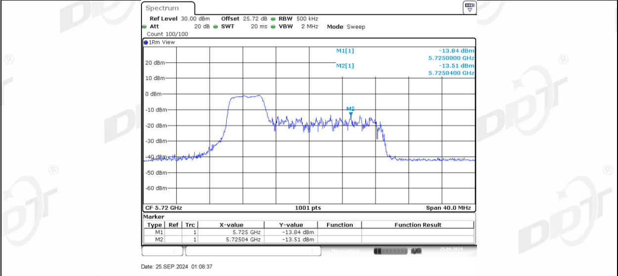
11AX20MIMO_Ant2_5720_UNII-3_52Tone_RU39
