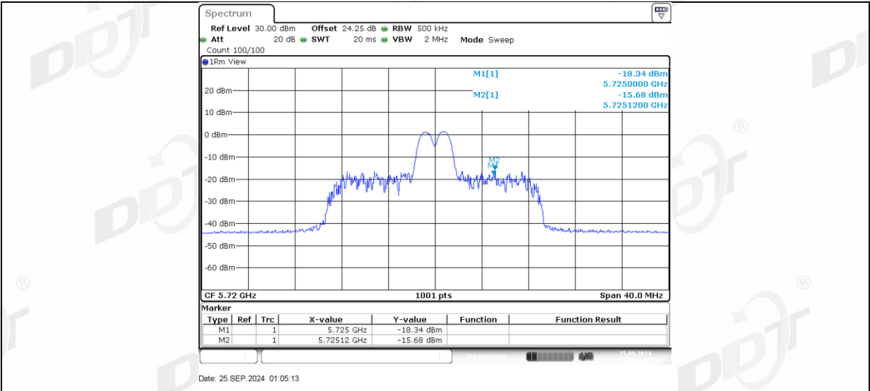
11AX20MIMO_Ant2_5720_UNII-3_26Tone_RU8
