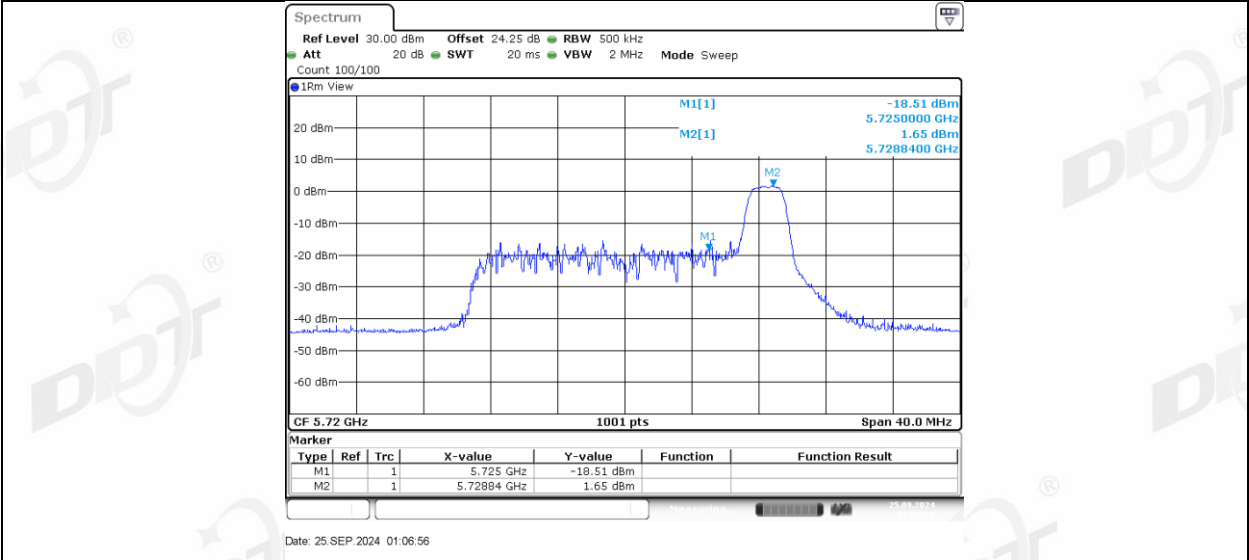
11AX20MIMO_Ant2_5720_UNII-3_52Tone_RU37
