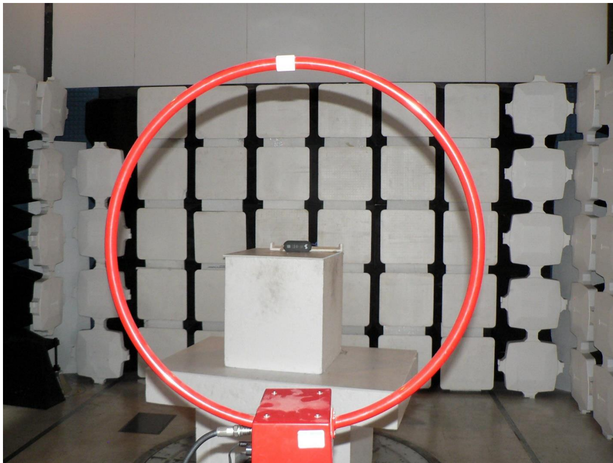
LYFT14 Scooter NFC 9KHz-30MHz
