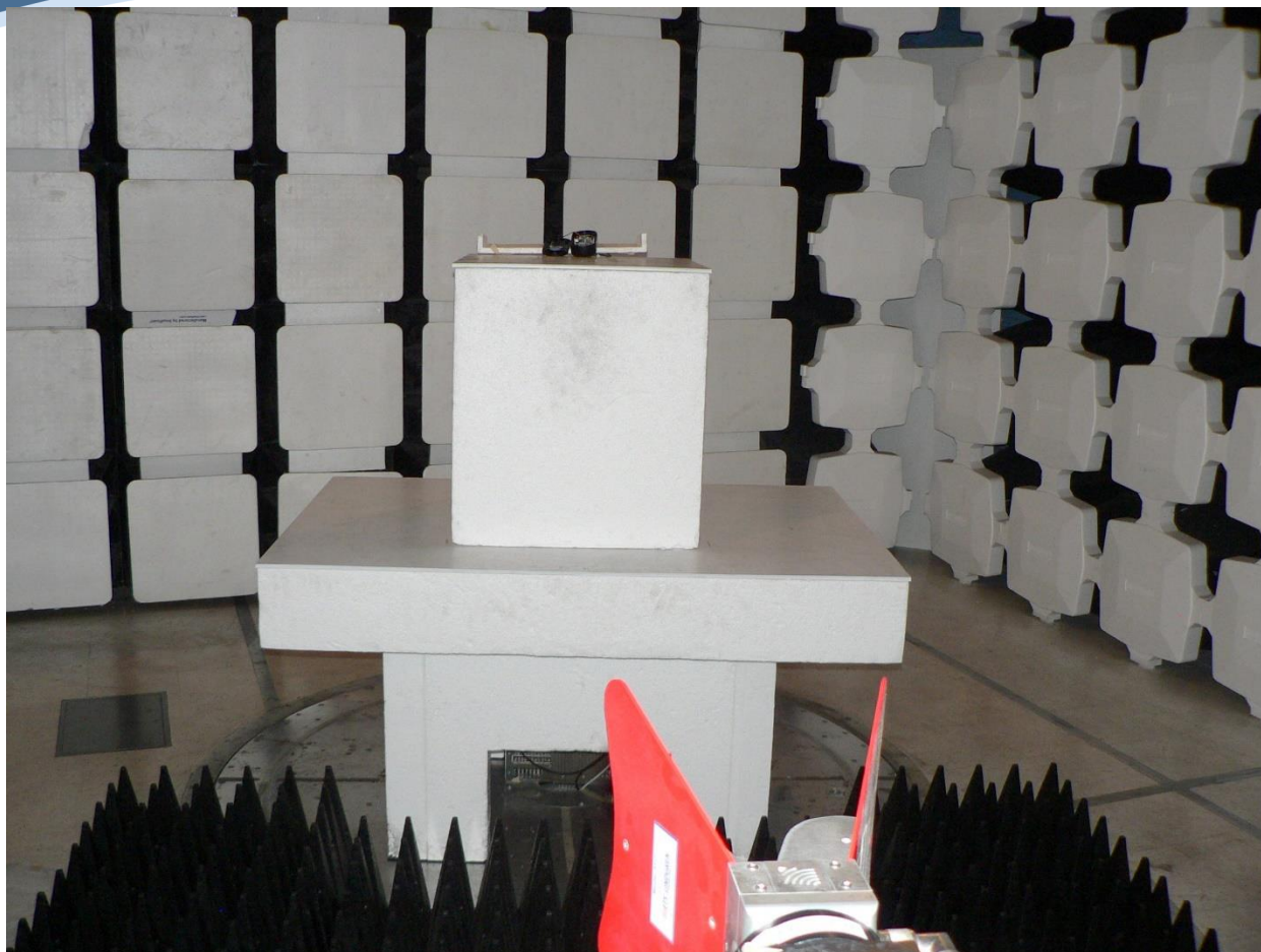
LYFT14 Scooter Tx Spurious 1-18GHz
