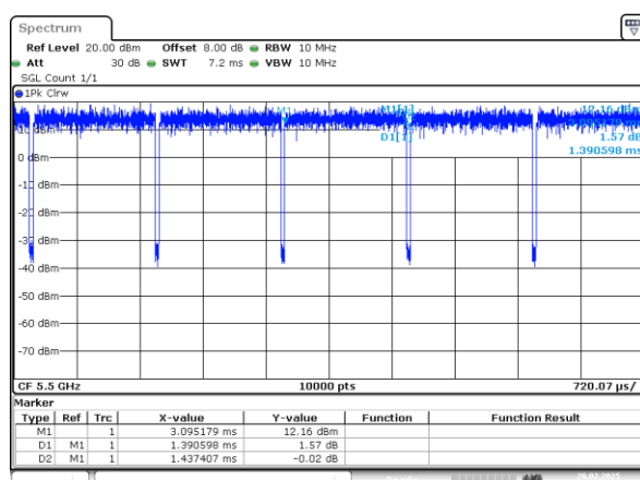
802.11a_5500MHz_Chain 1
