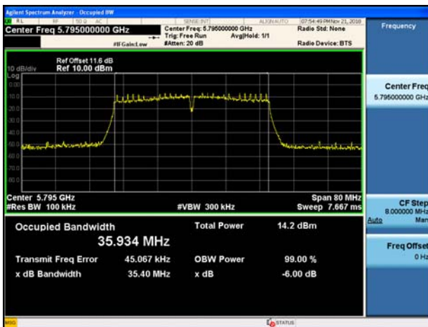
802.11n(HT40) (CH.159)
