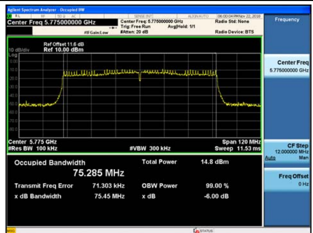
802.11ac(VHT80) (CH.155)
