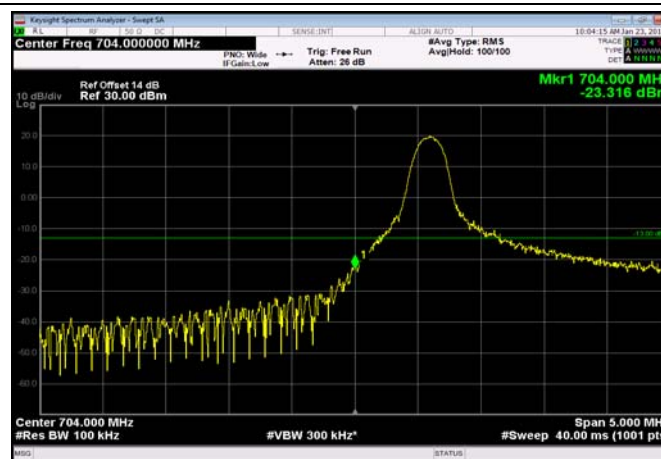
LowRange_FDD17_10MHz_709_OneRB _low_Q16
