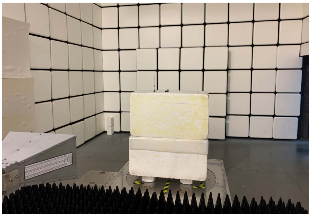
1GHz-18GHz
