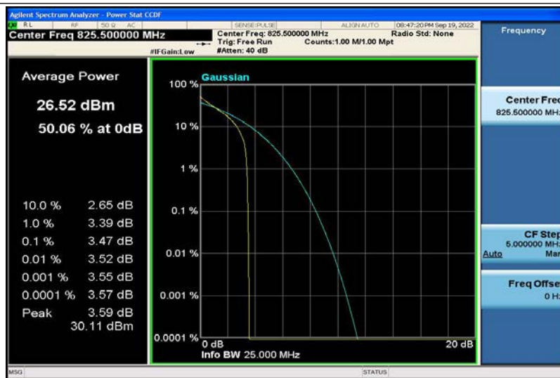
Band5-3MHz-QPSK-20415-1RB#0
