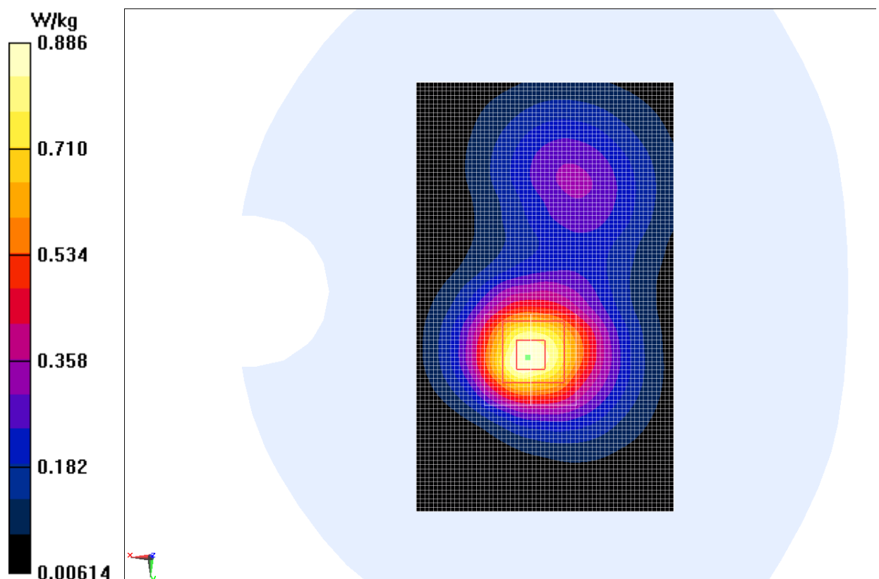
Fig.I.8 WCDMA1900 CH9262
