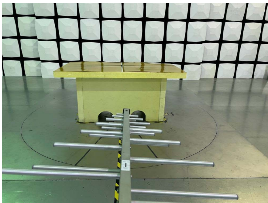
Below 1GHz(BLE)
