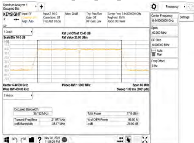
802.11n_40MHz_Chain3_6445MHz
