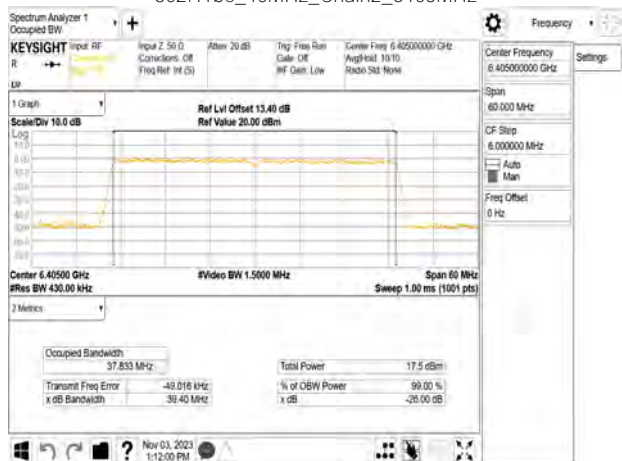
802.11be_40MHz_Chain2_6405MHz
