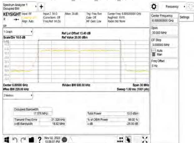
802.11n_20MHz_Chain0_6895MHz
