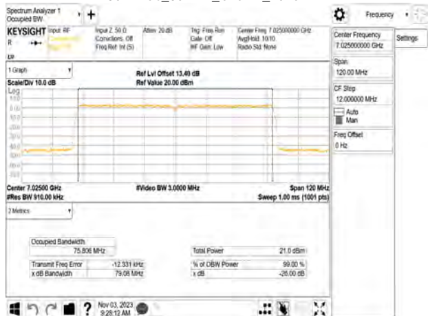
802.11ac_80MHz_Chain2_7025MHz
