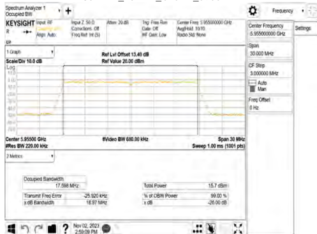
802.11n_20MHz_Chain1_5955MHz
