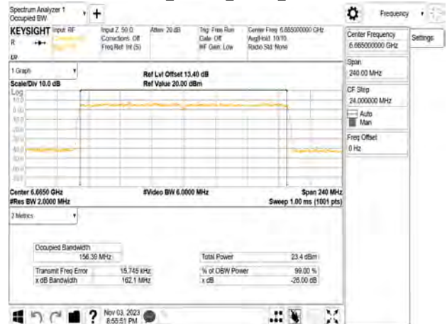
802.11be_160MHz_Chain3_6665MHz
