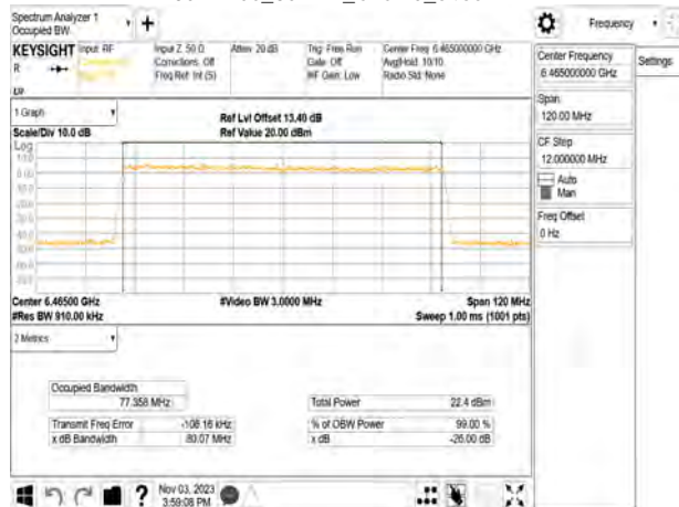
802.11be_80MHz_Chain0_6465MHz
