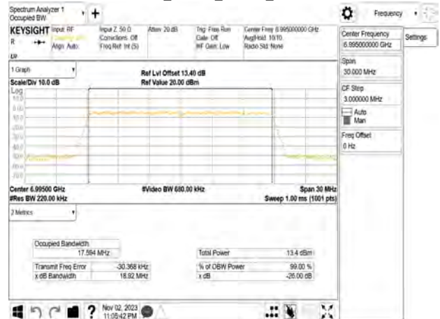
802.11n_20MHz_Chain2_6995MHz
