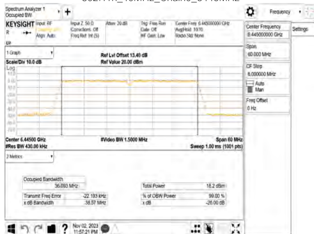
802.11n_40MHz_Chain0_6445MHz
