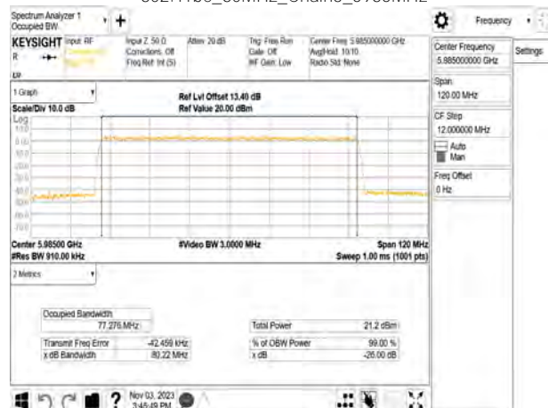
802.11be_80MHz_Chain3_5985MHz
