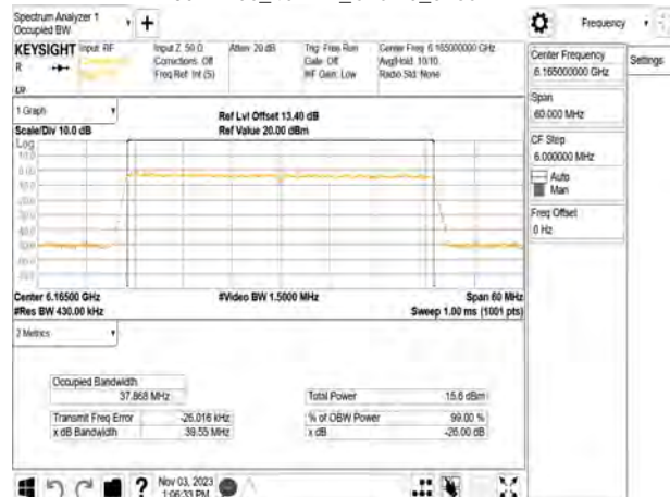
802.11be_40MHz_Chain0_6165MHz
