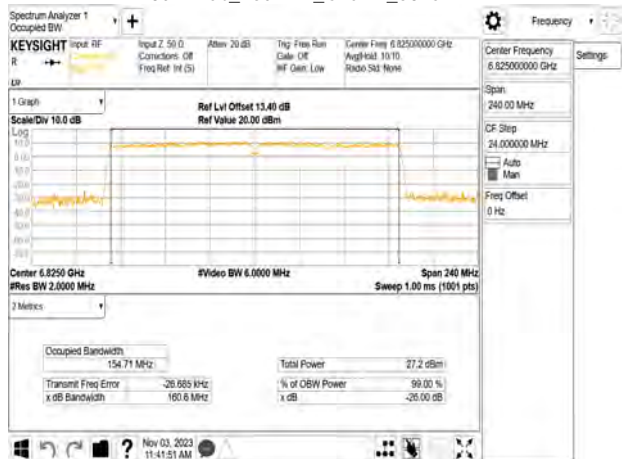
802.11ac_160MHz_Chain1_6825MHz
