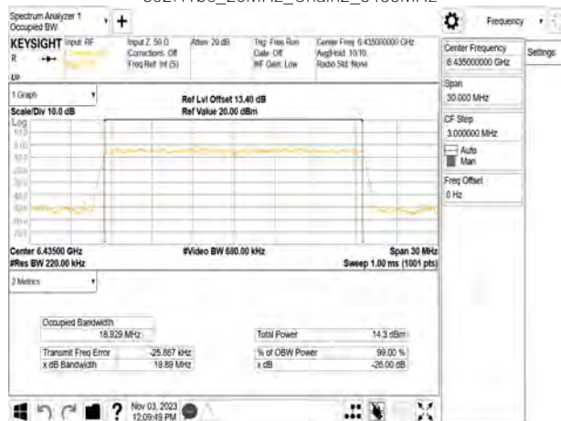
802.11be_20MHz_Chain2_6435MHz
