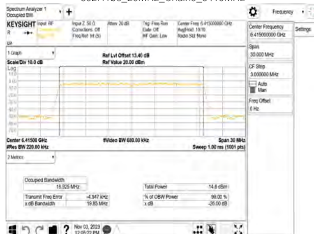
802.11be_20MHz_Chain3_6415MHz
