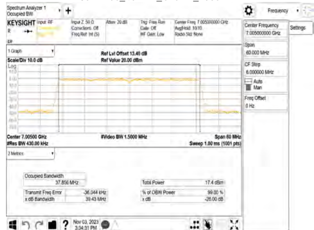
802.11be_40MHz_Chain2_7005MHz
