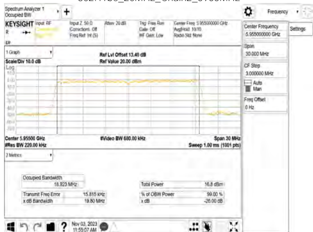
802.11be_20MHz_Chain2_5955MHz
