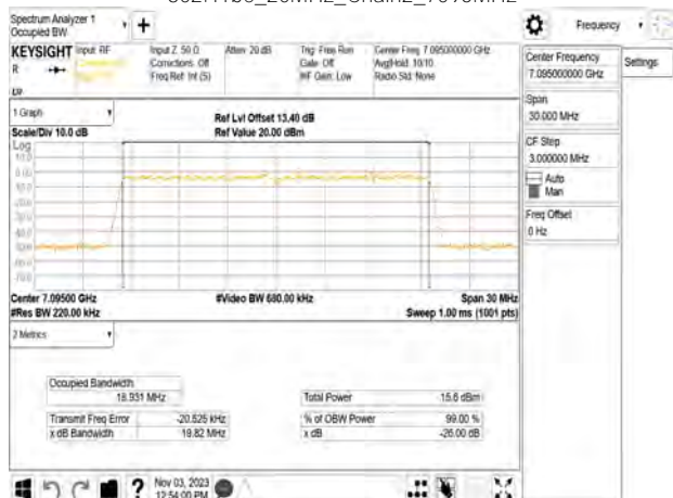
802.11be_20MHz_Chain2_7095MHz
