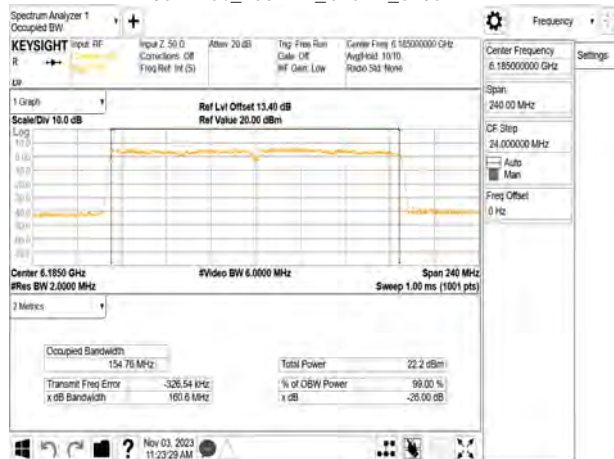
802.11ac_160MHz_Chain2_6185MHz
