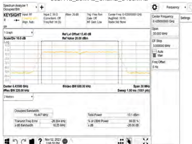
802.11a_20MHz_Chain2_6435MHz
