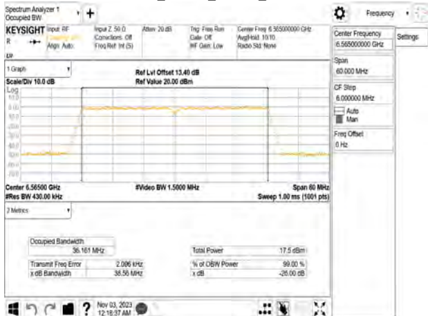
802.11n_40MHz_Chain0_6565MHz
