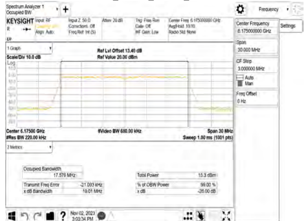
802.11n_20MHz_Chain0_6175MHz
