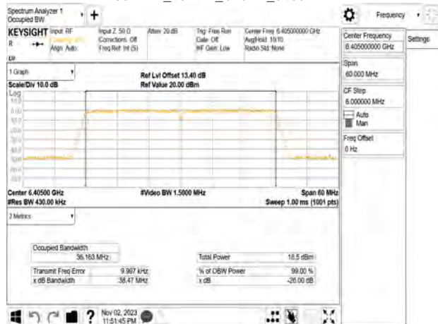
802.11n_40MHz_Chain1_6405MHz
