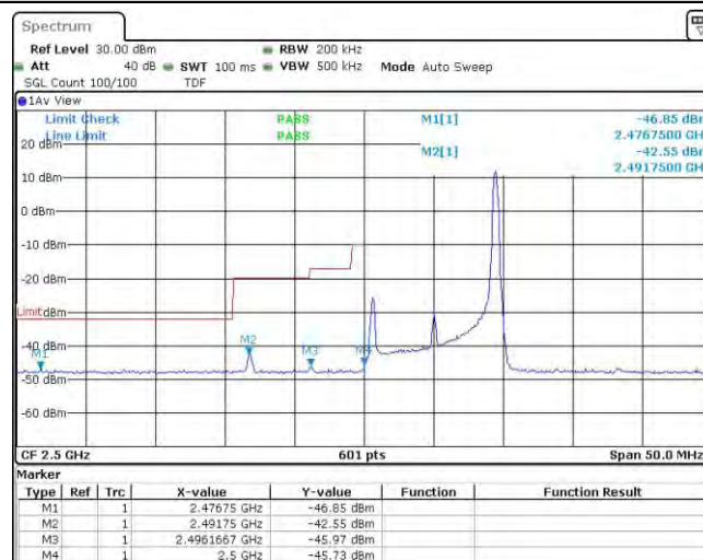
Band7-10MHz-QPSK-20800-50RB#0
