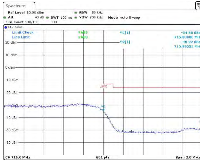
Band12-3MHz-QPSK-23165-1RB#14
