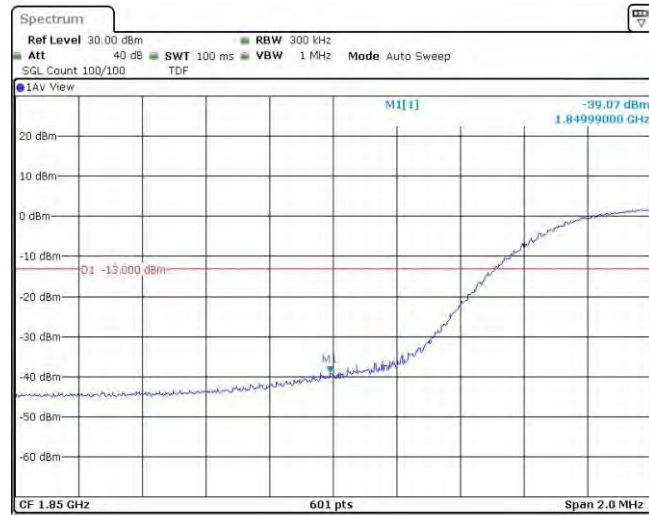
Band2-15MHz-QPSK-18675-1RB#74
